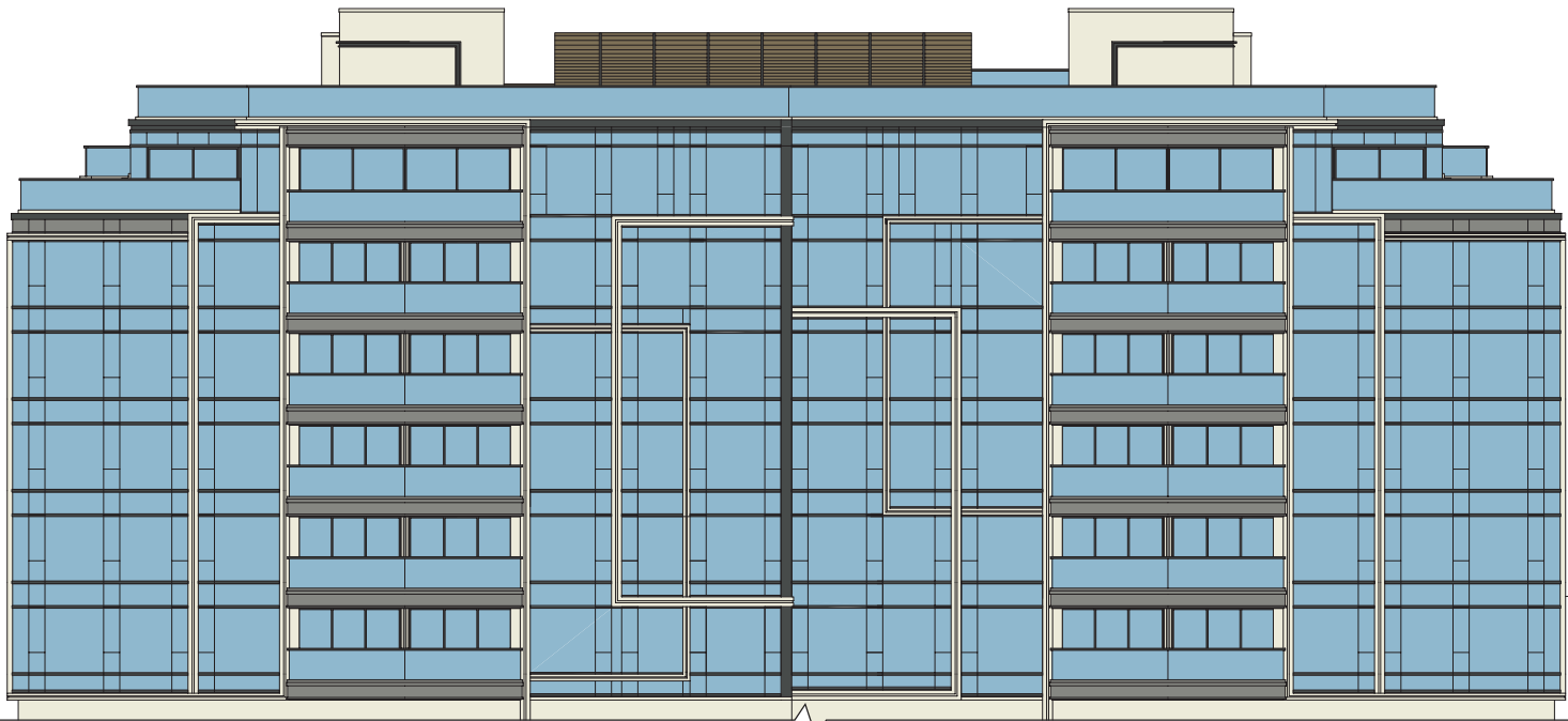
ELEVATION E 立面 E
