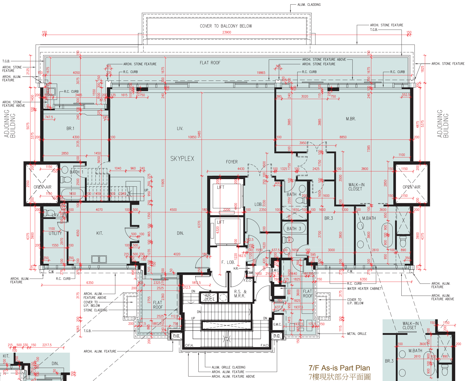
7/F As-is Part Plan 7樓現狀部分平面圖
