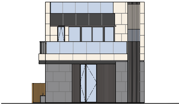
Elevation Plan 6 立面圖六
