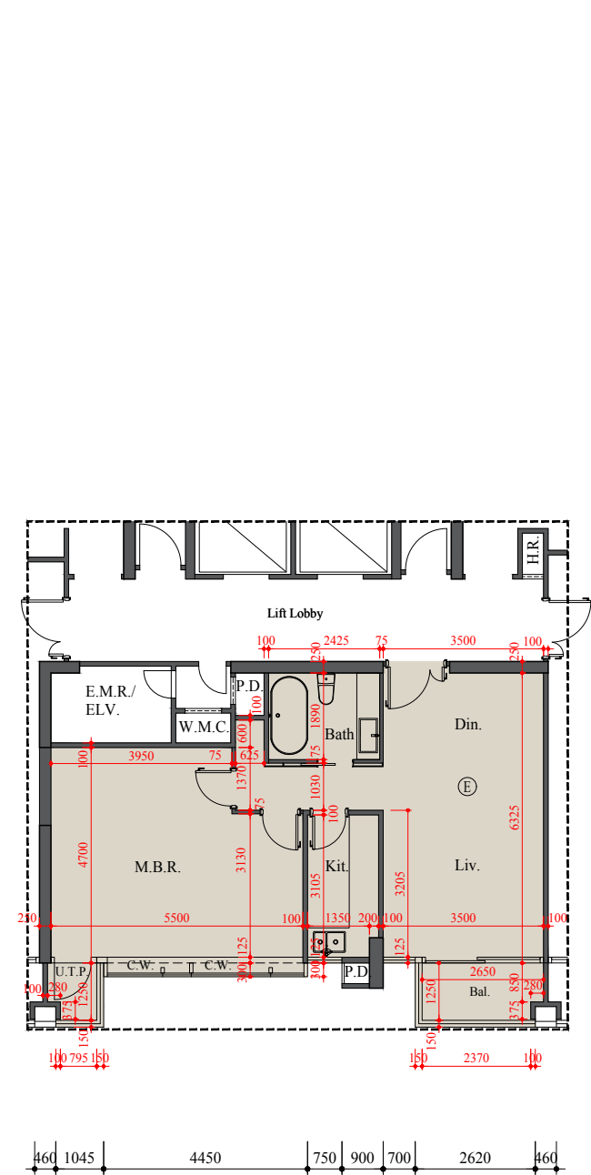
Block 5 5 座 Part Plan of 16/F (Flat E) 16樓(單位E)之部份平面圖
