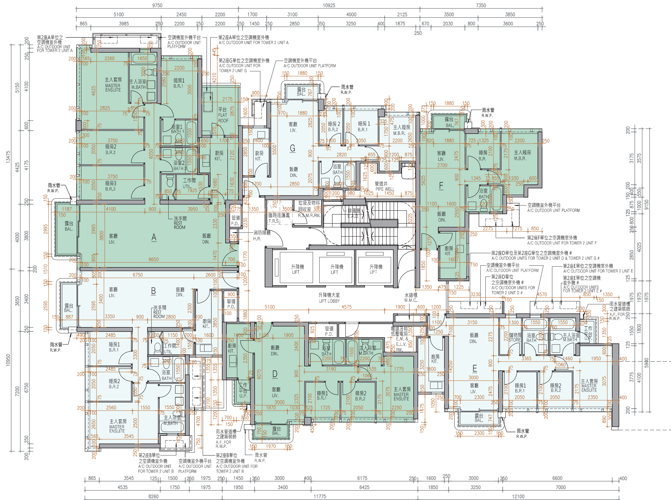
TOWER 2 3/F FLOOR PLAN 第2座 3樓 樓面平面圖
