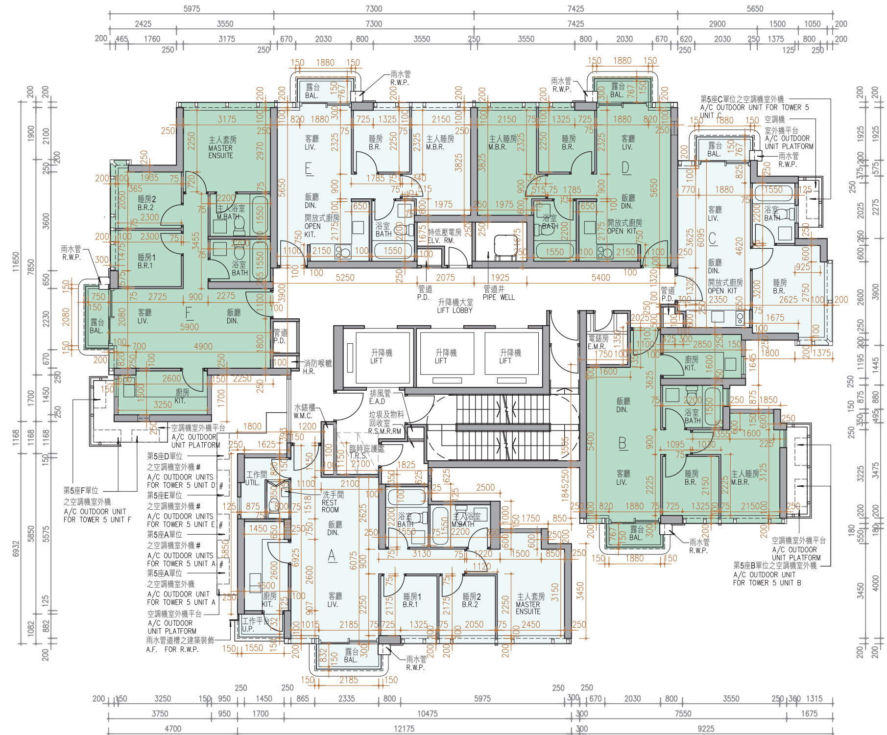
TOWER 5 6/F-12/F & 15/F-20/F FLOOR PLAN 第5座 6樓至12樓及15樓至20樓 樓面平面圖
