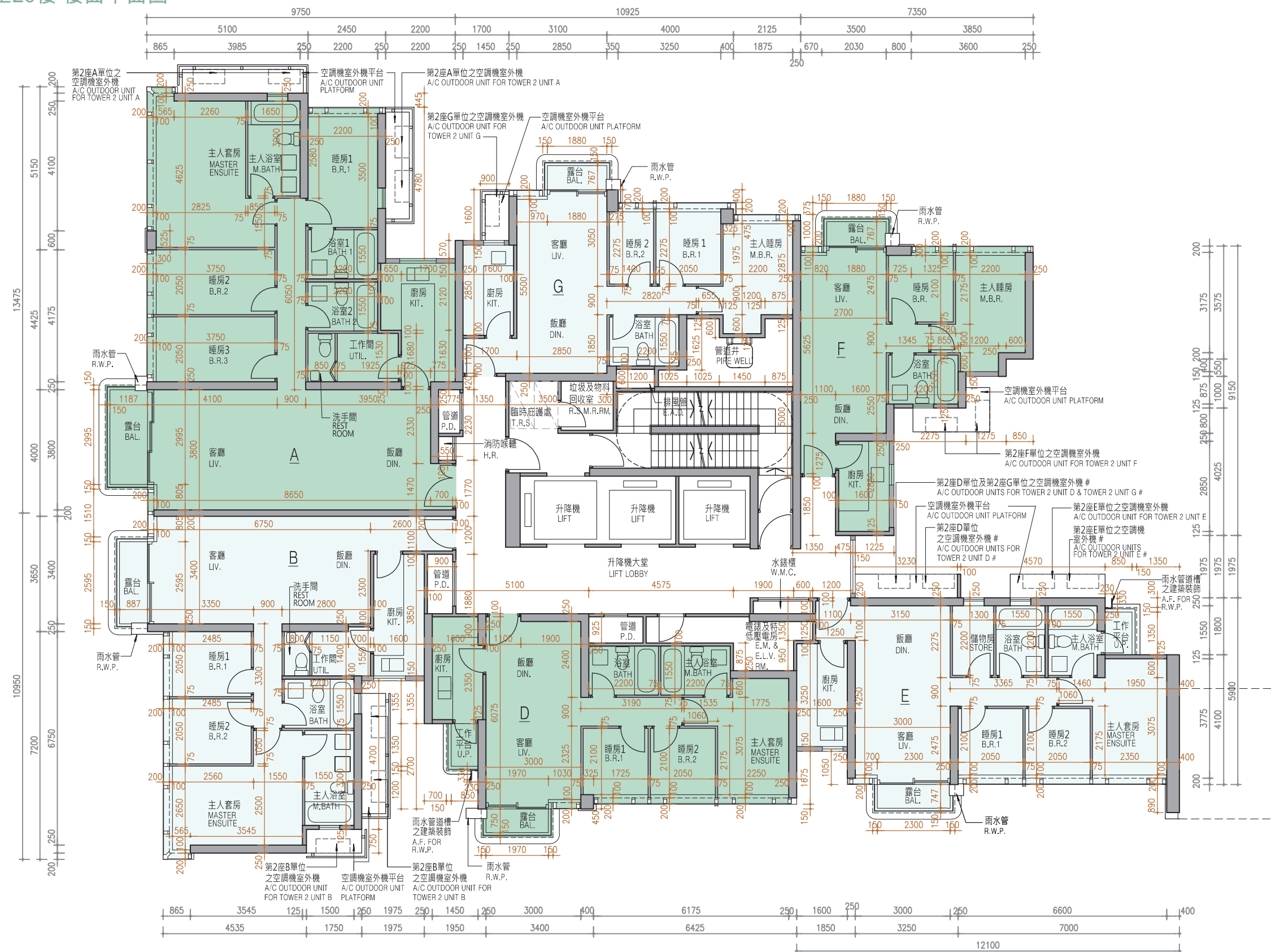
TOWER 2 19/F-20/F FLOOR PLAN 第2座 19樓至20樓 樓面平面圖
