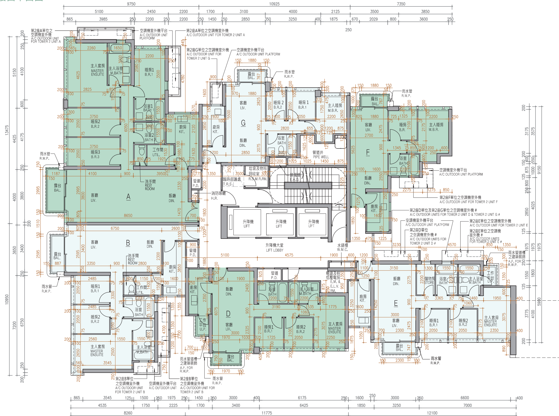
TOWER 2 22/F FLOOR PLAN 第2座 22樓 樓面平面圖
