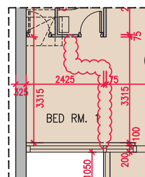
Part Plan of lower part of Tower 1 (1A) Unit C on 35/F 第1座(1A)35樓C單位下層之部份圖
