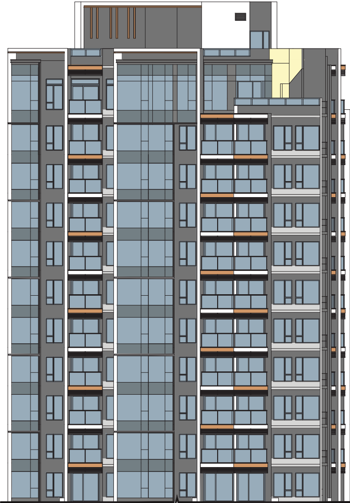
ELEVATION 2 立面 2
