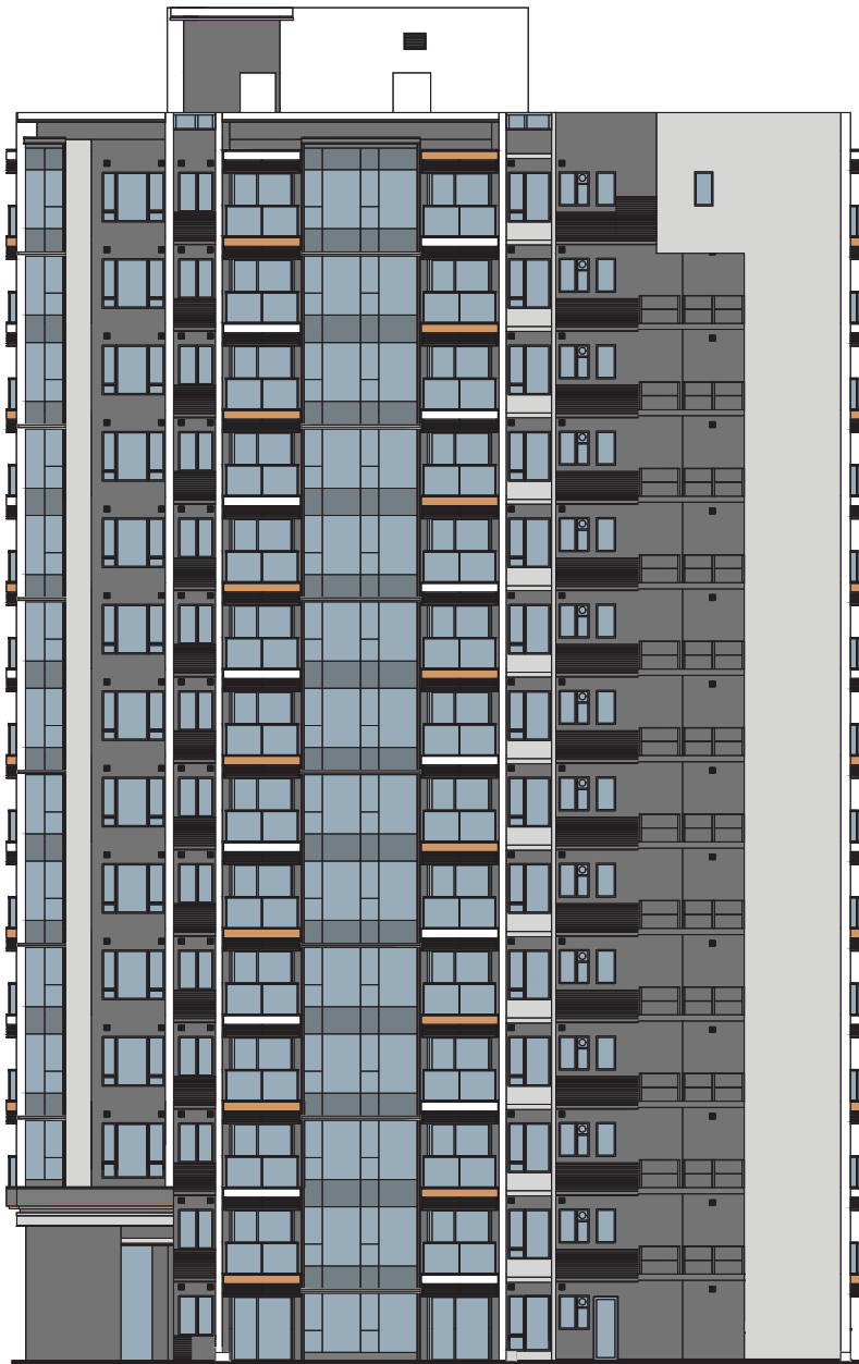
ELEVATION 3 立面 3
