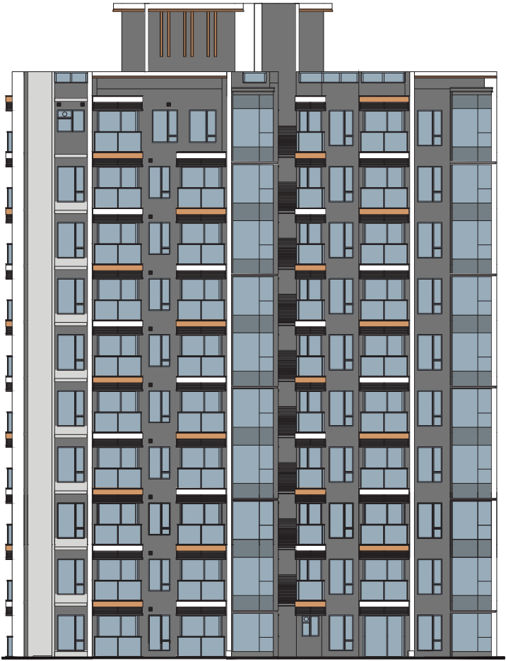
ELEVATION 4 立面 4
