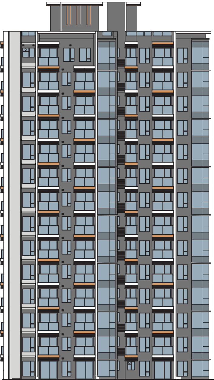
ELEVATION 4 立面 4
