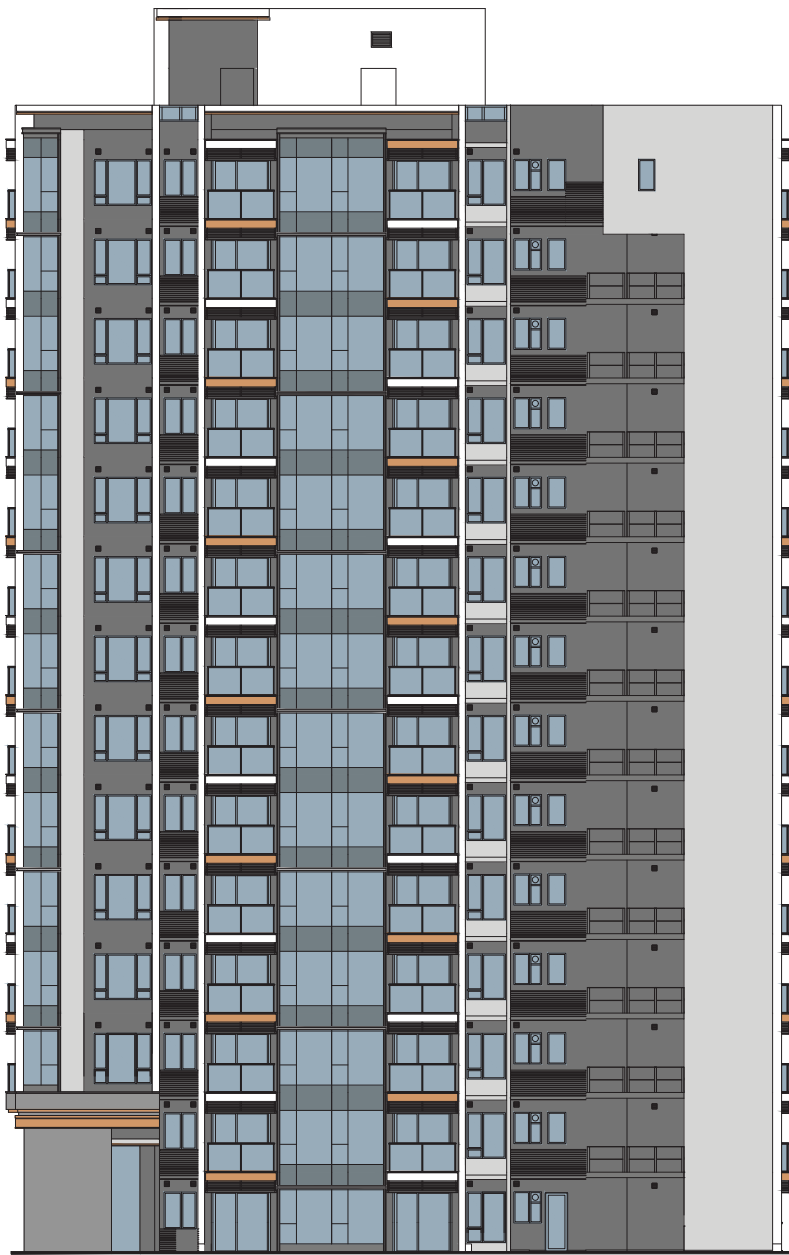
ELEVATION 3 立面 3
