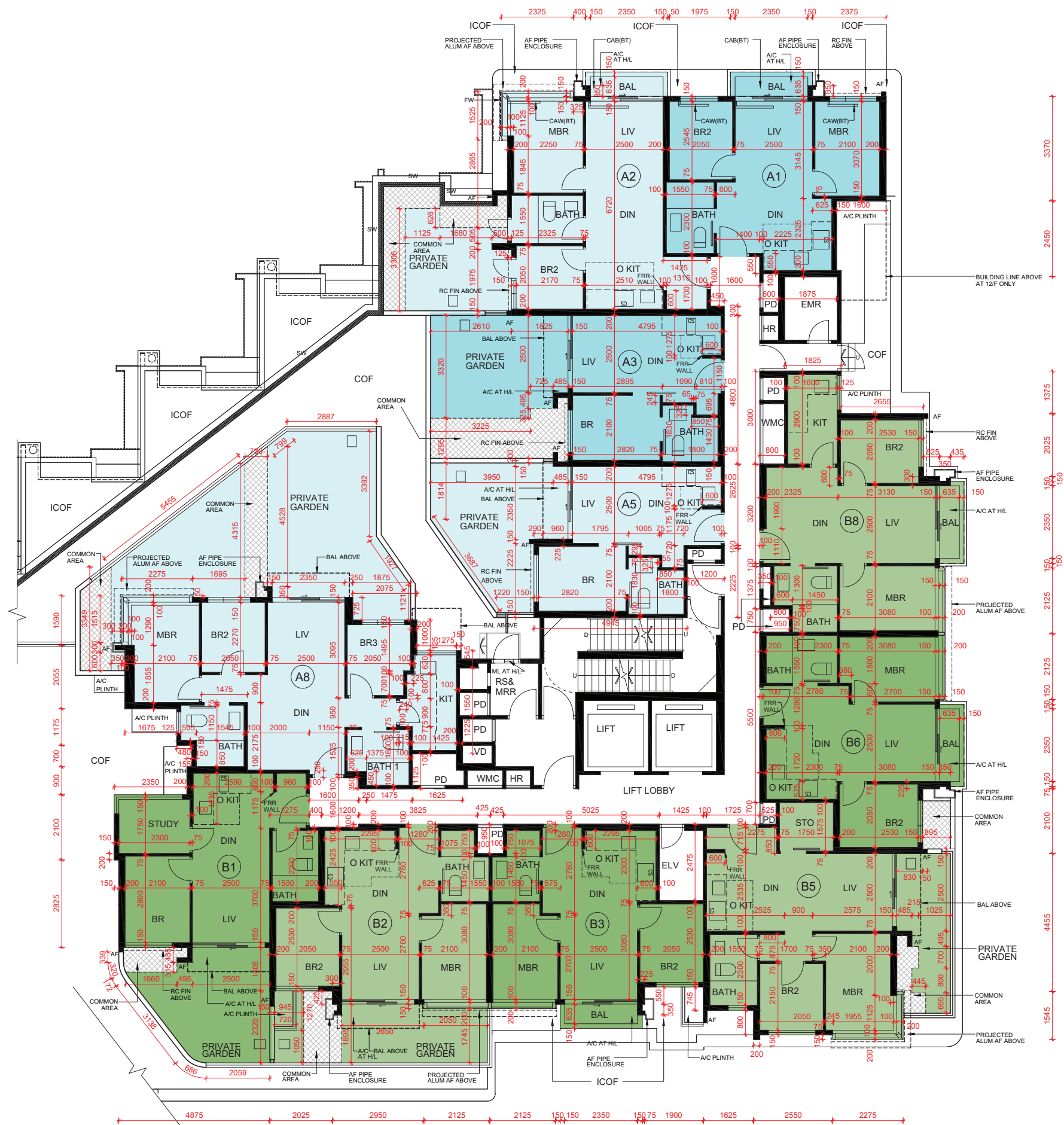
SCENIC TOWER 5 3/F FLOOR PLAN 優景閣第5座 3樓平面圖
