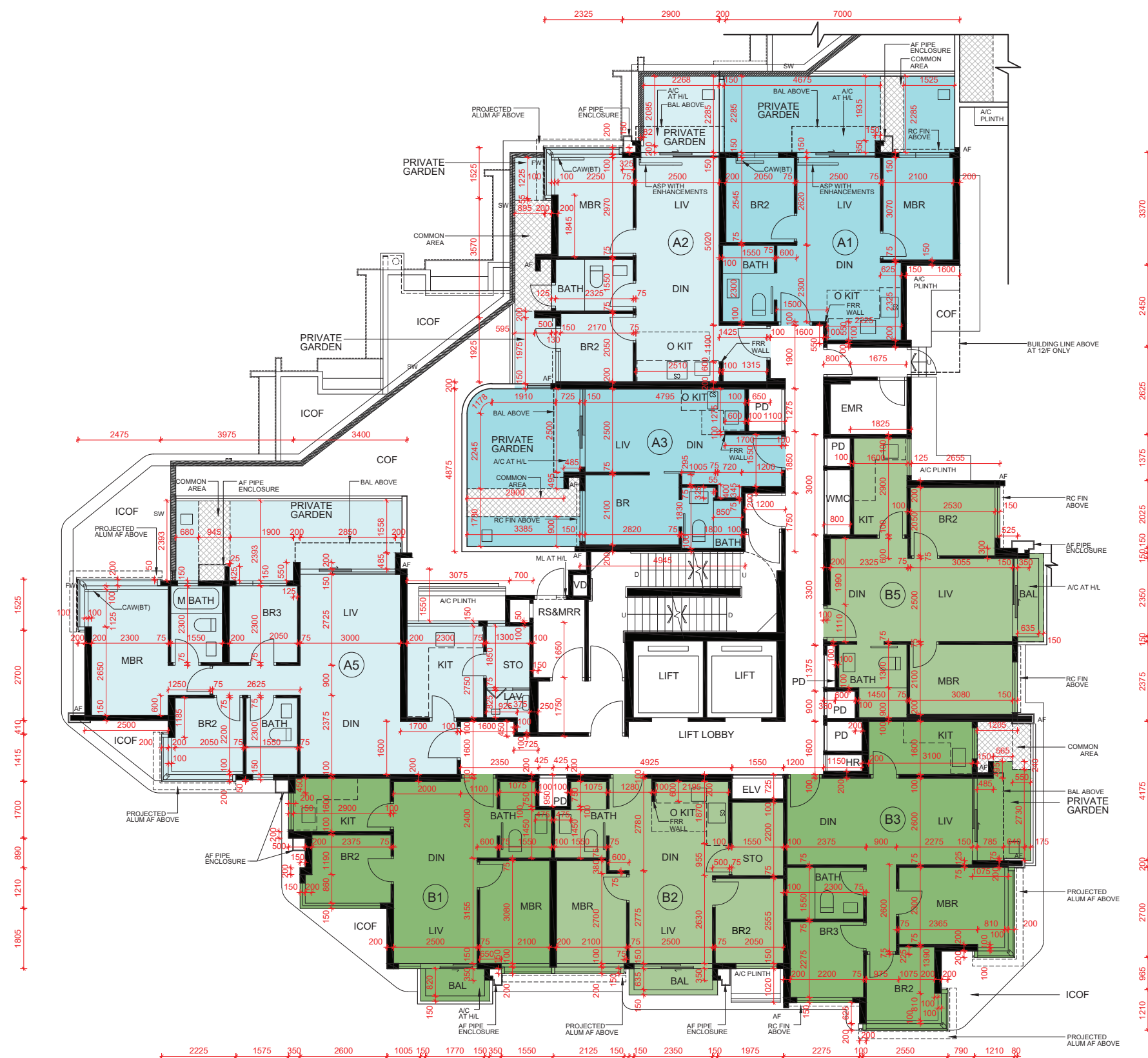
SCENIC TOWER 6 3/F FLOOR PLAN 優景閣第6座 3樓平面圖
