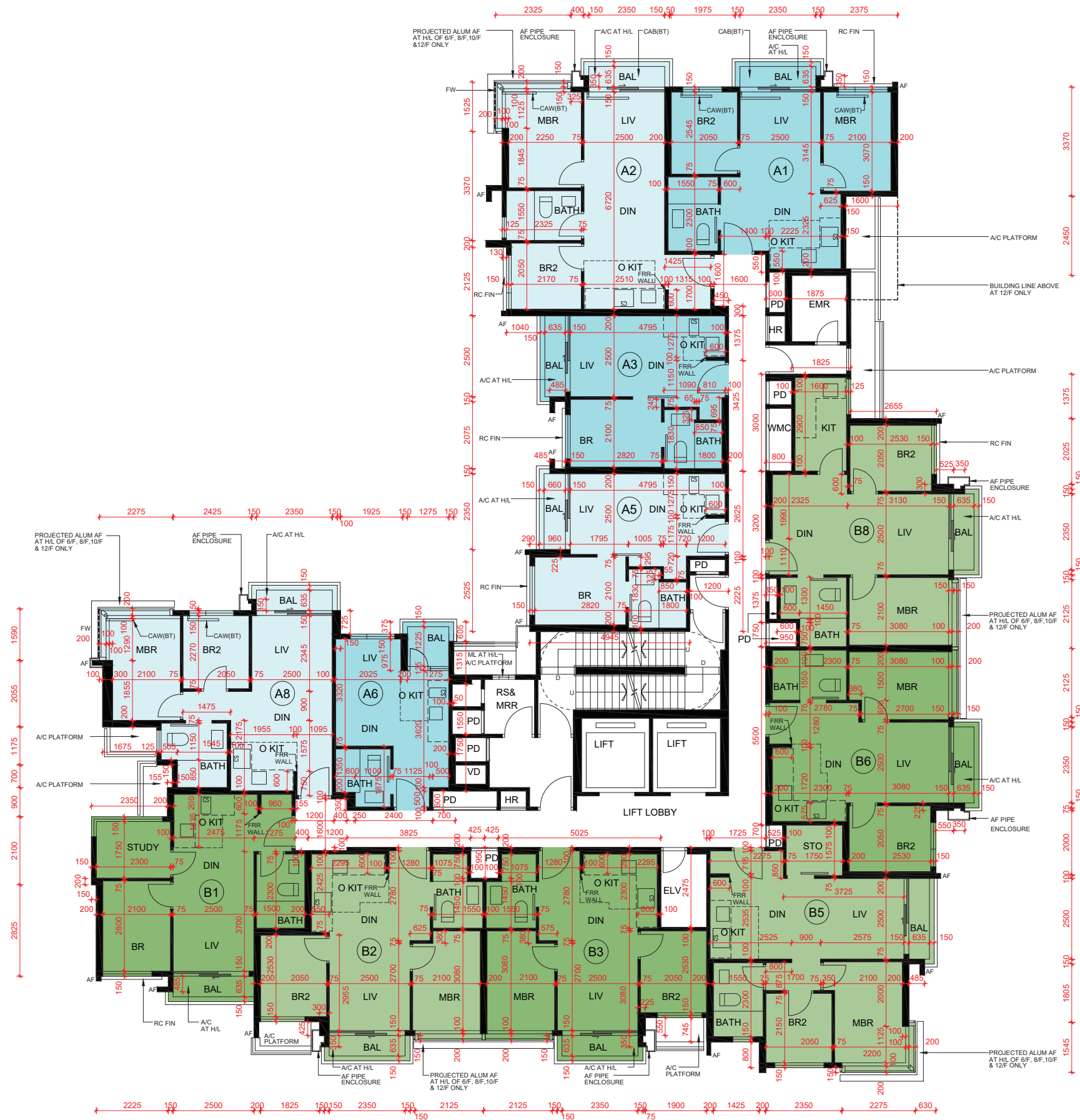
SCENIC TOWER 5 5/F-12/F FLOOR PLAN 優景閣第5座 5樓至12樓平面圖
