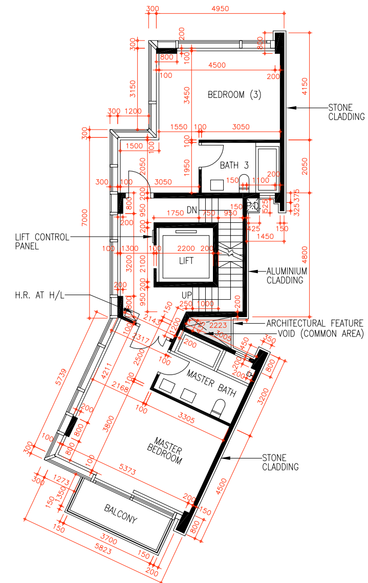
SECOND FLOOR PLAN 二樓平面圖
