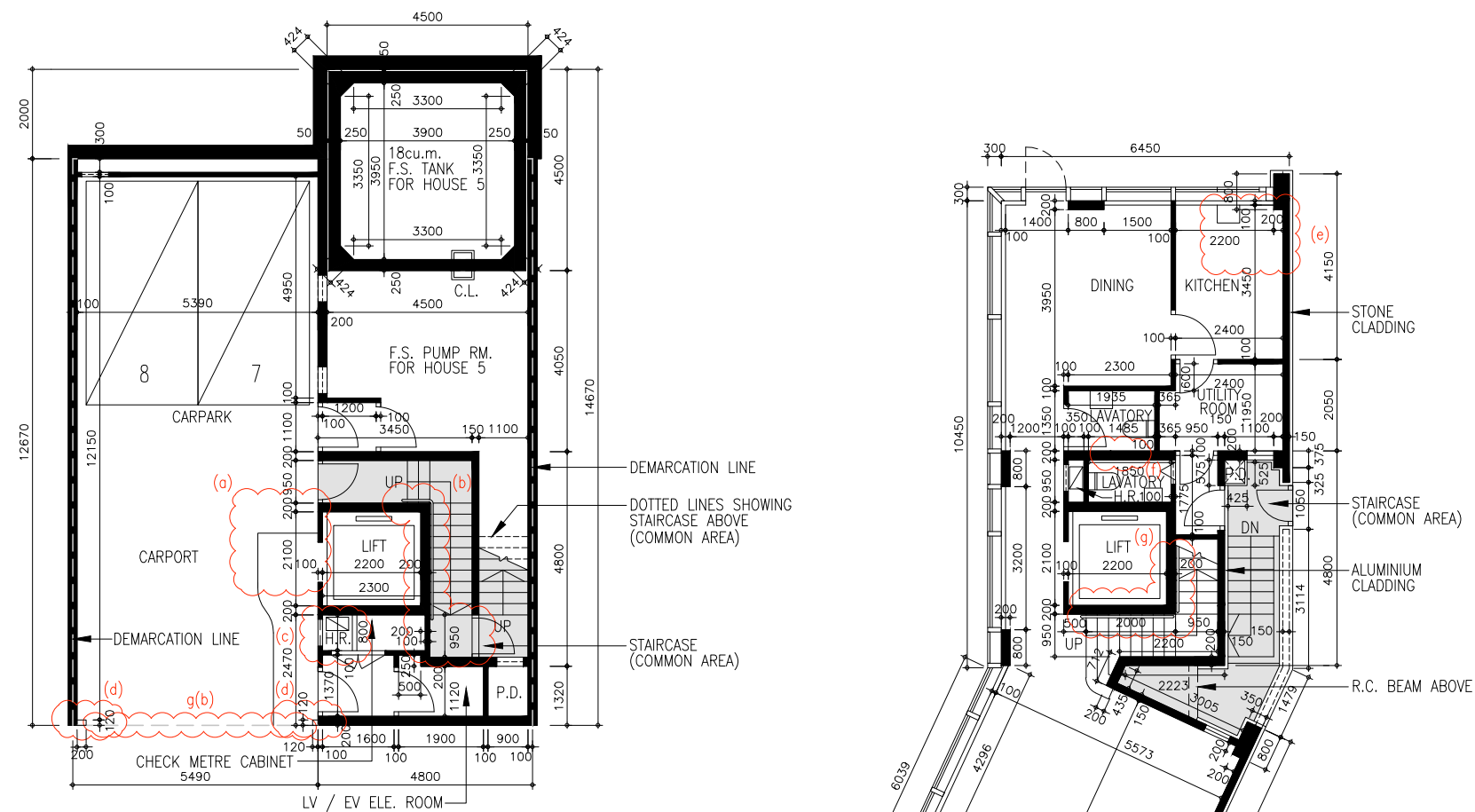
LOWER GROUND FLOOR PLAN 地下低層平面圖
