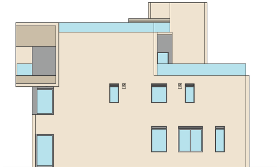
ELEVATION 4 立面圖 4
