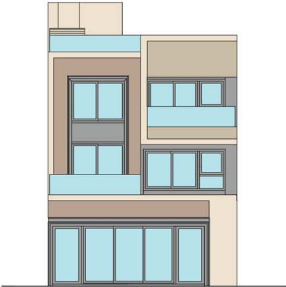
ELEVATION 1 立面圖 1
