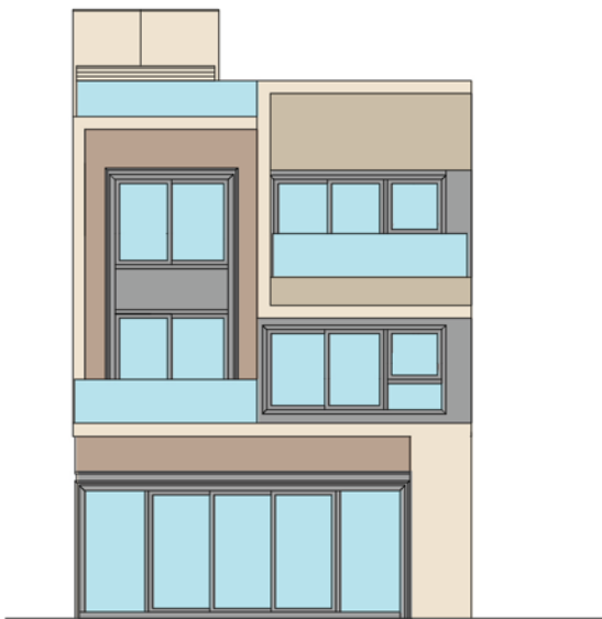
ELEVATION 1 立面圖 1
