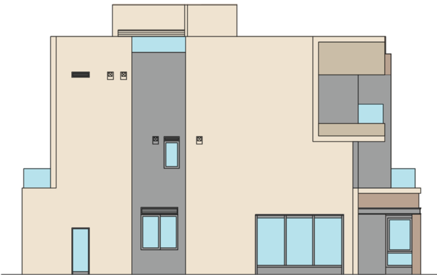
ELEVATION 2 立面圖 2
