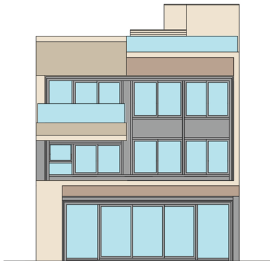
ELEVATION 1 立面圖 1
