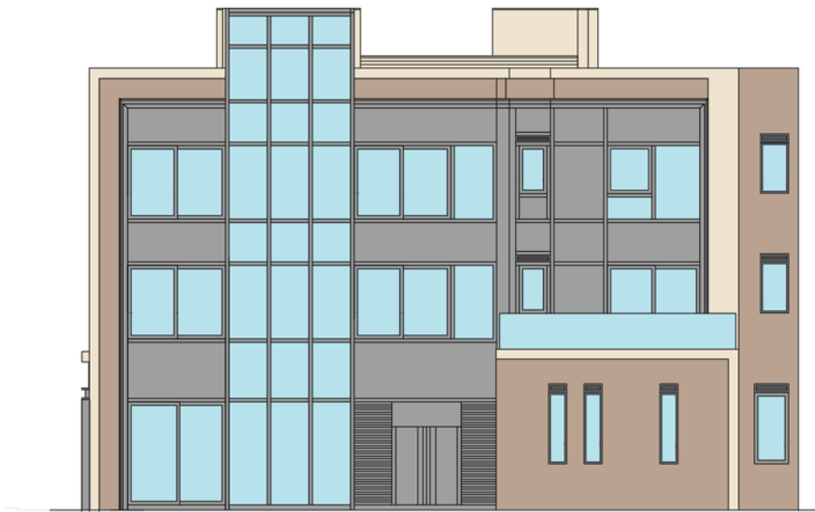
ELEVATION 3 立面圖 3
