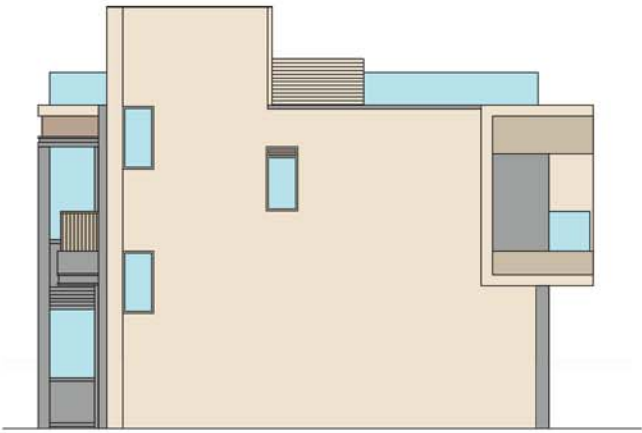
ELEVATION 2 立面圖 2
