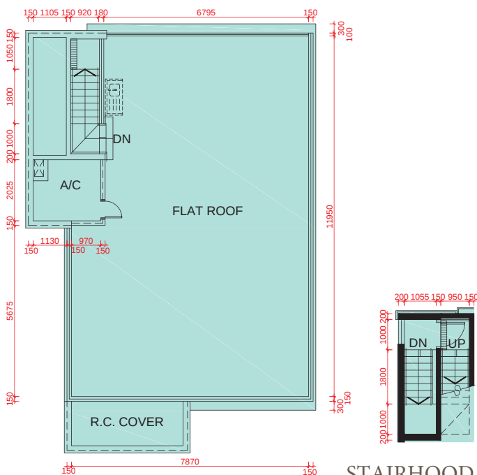
STAIRHOOD PLAN 梯屋平面圖
