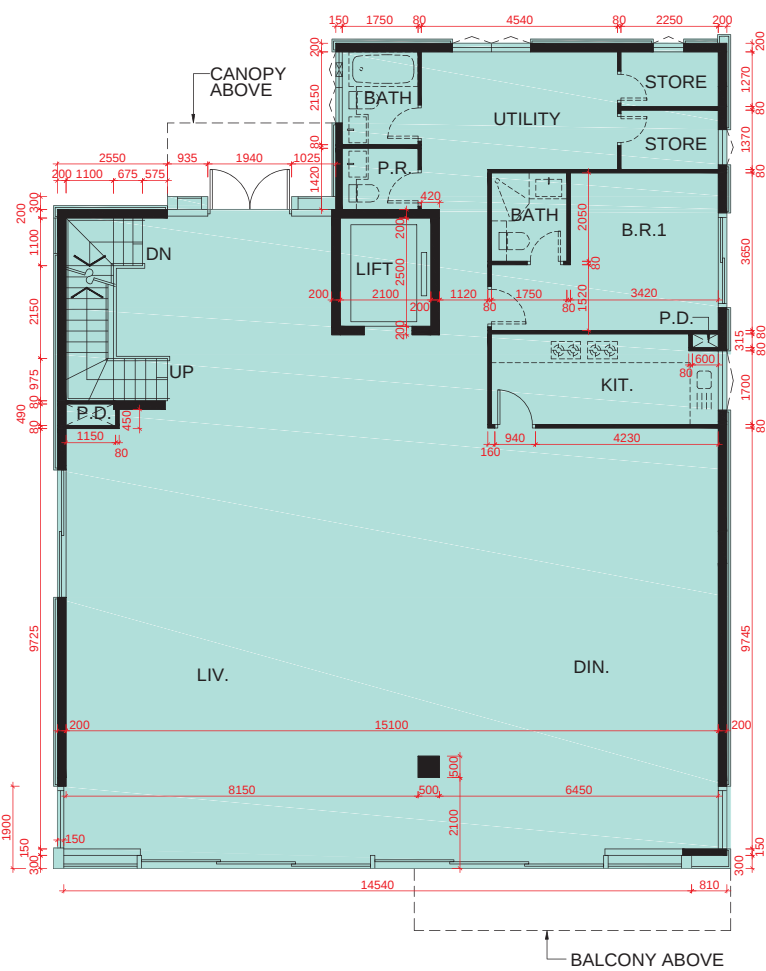
G/F PLAN 地面層平面圖
