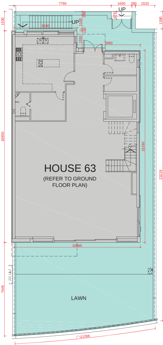
G/F PLAN (FOR GARDEN) 地面層平面圖 (花園)
