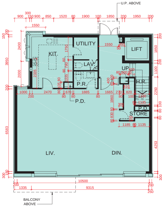
G/F PLAN 地面層平面圖
