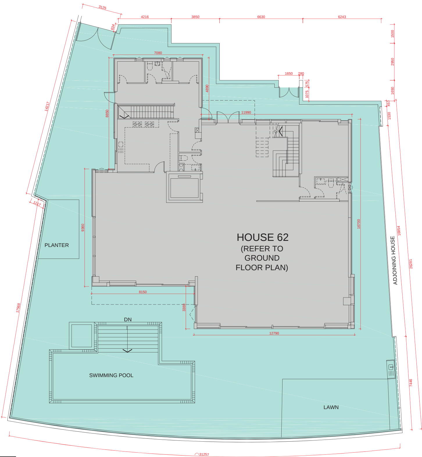
G/F PLAN (FOR GARDEN) 地面層平面圖 (花園)
