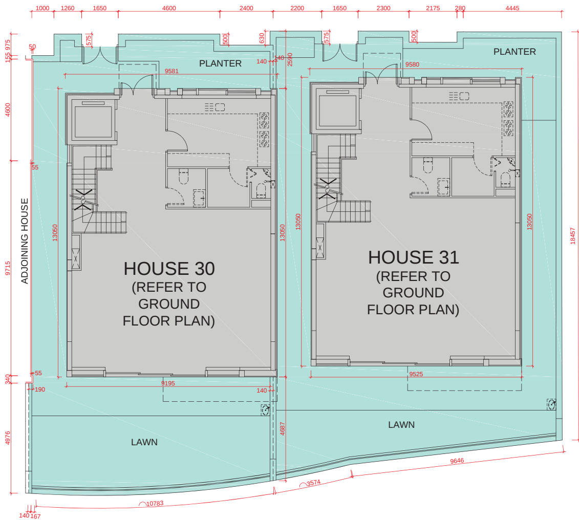
G/F PLAN (FOR GARDEN) 地面層平面圖 (花園)
