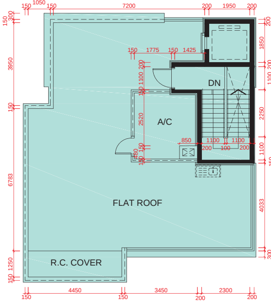
ROOF PLAN 天台平面圖
