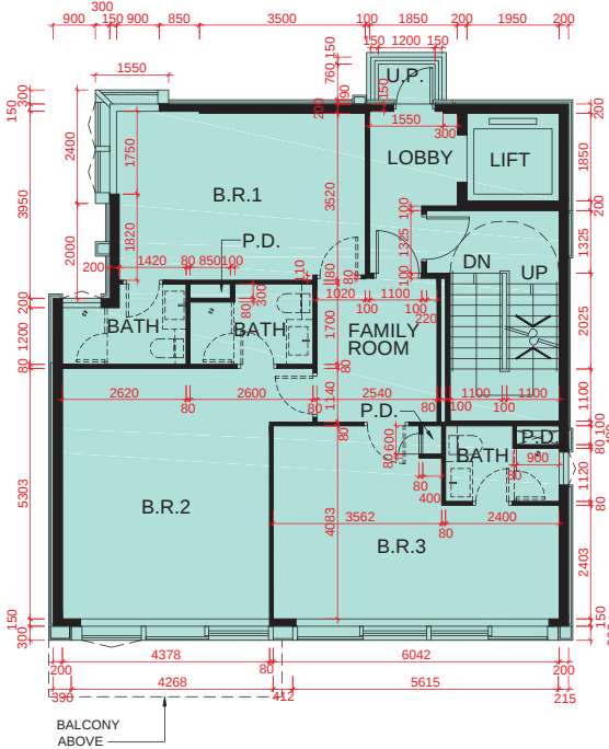
1/F PLAN 1樓平面圖
