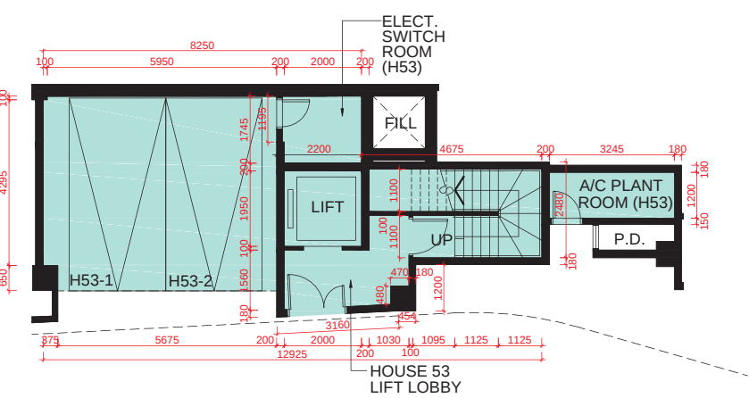
B/F PLAN 地庫層平面圖
