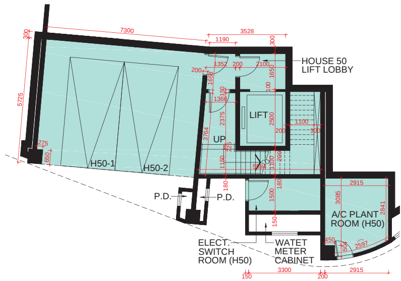
B/F PLAN 地庫層平面圖
