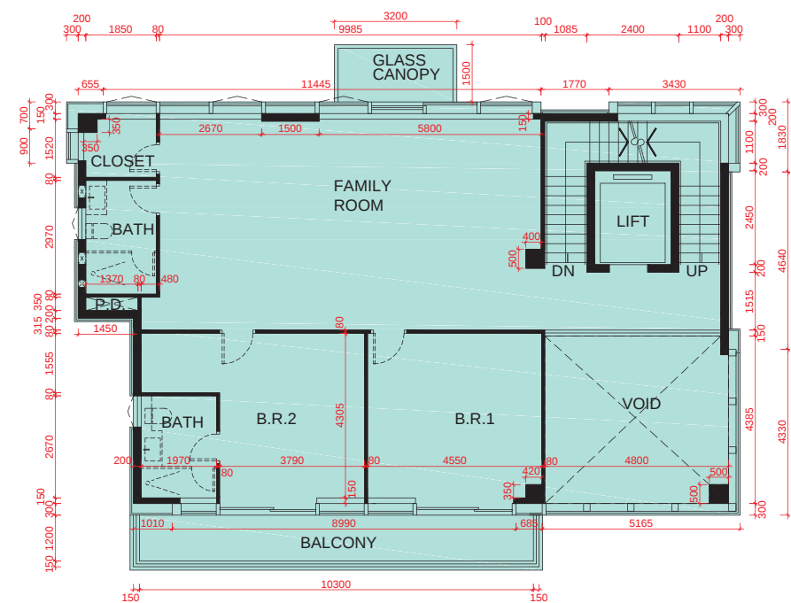
1/F PLAN 1樓平面圖
