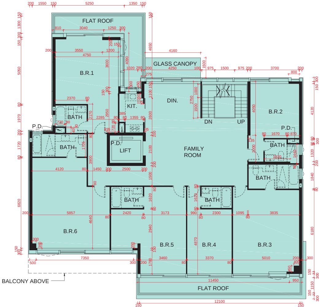
1/F PLAN 1樓平面圖
