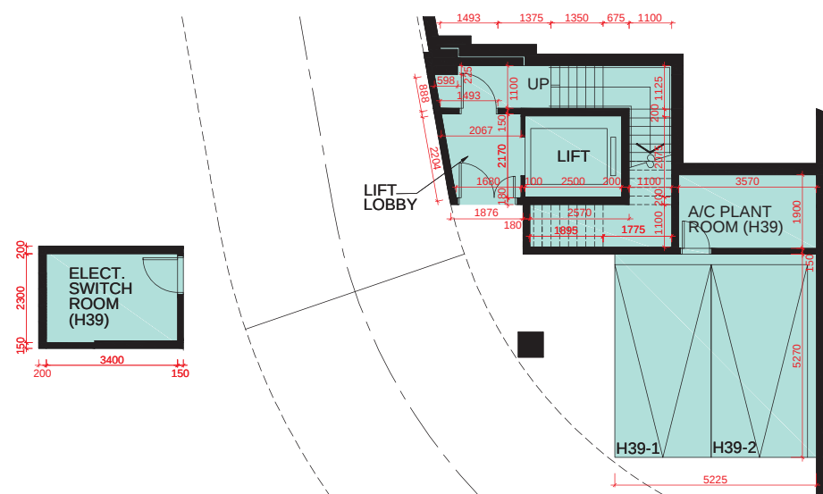
B/F PLAN 地庫層平面圖
