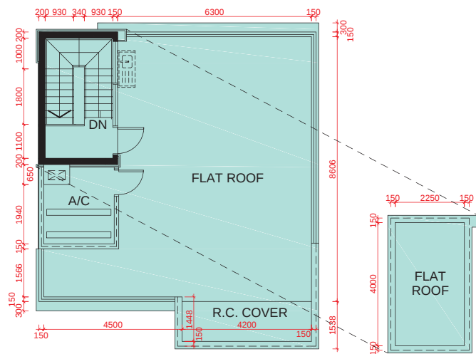
UPPER ROOF PLAN 上層天台平面圖
