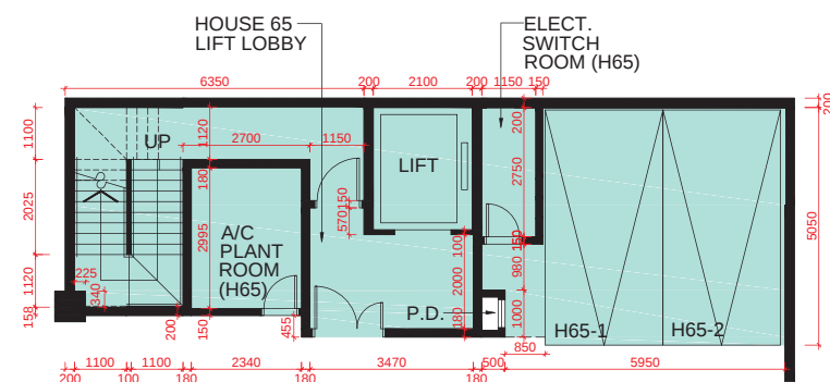
B/F PLAN 地庫層平面圖
