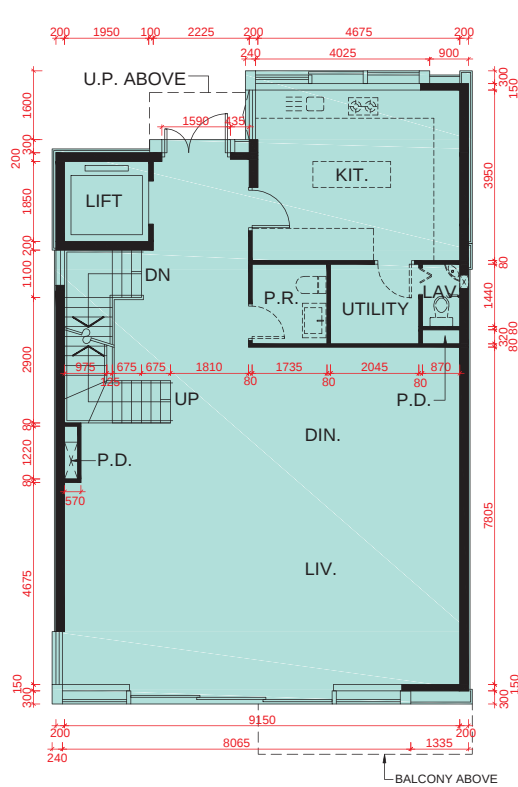
G/F PLAN 地面層平面圖
