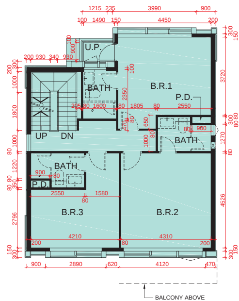
1/F PLAN 1樓平面圖
