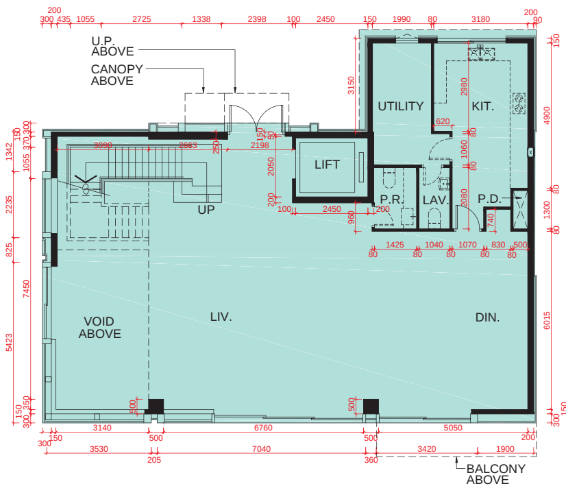
G/F PLAN 地面層平面圖
