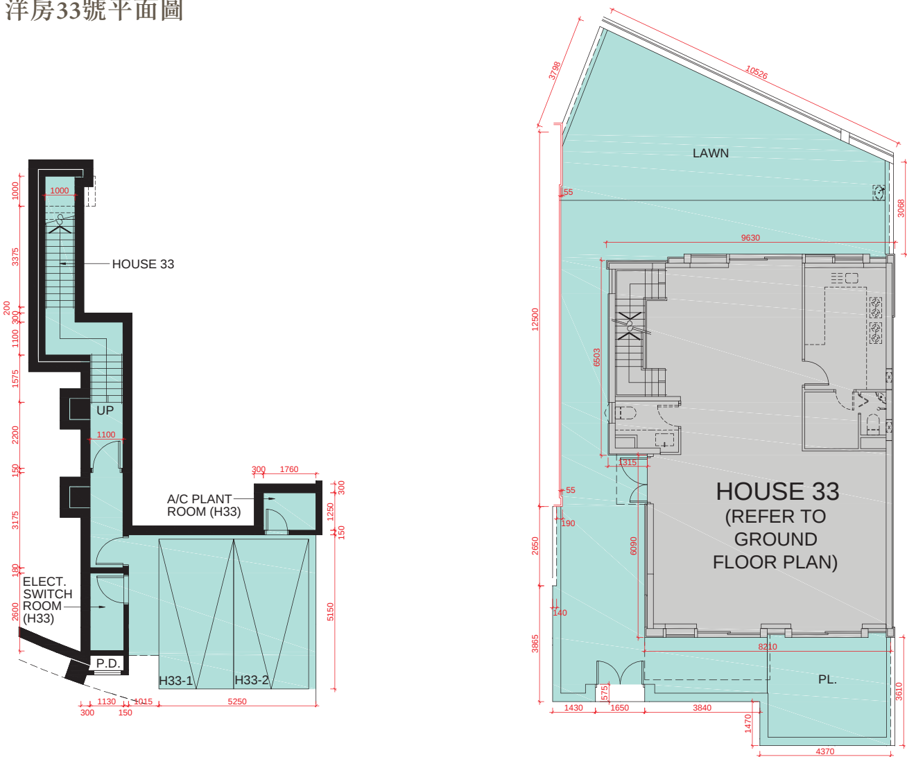
B/F PLAN 地庫層平面圖
