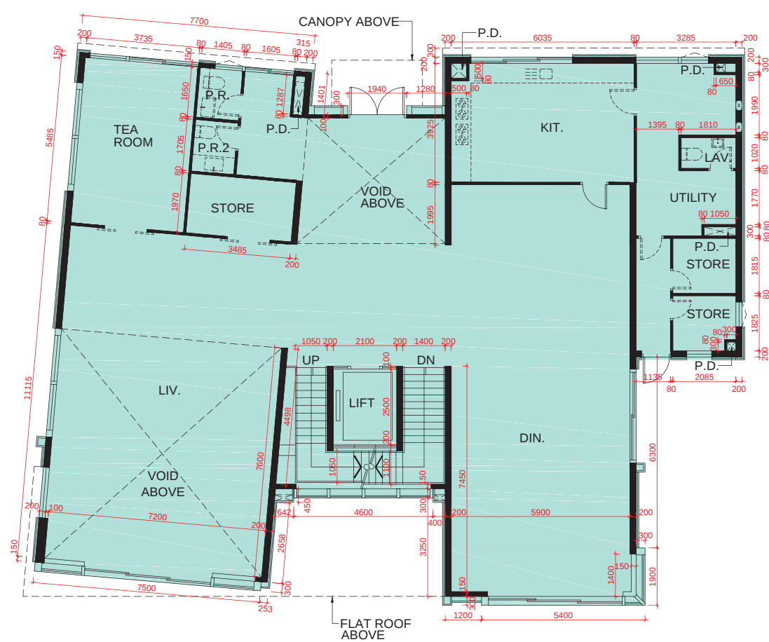
G/F PLAN 地面層平面圖
