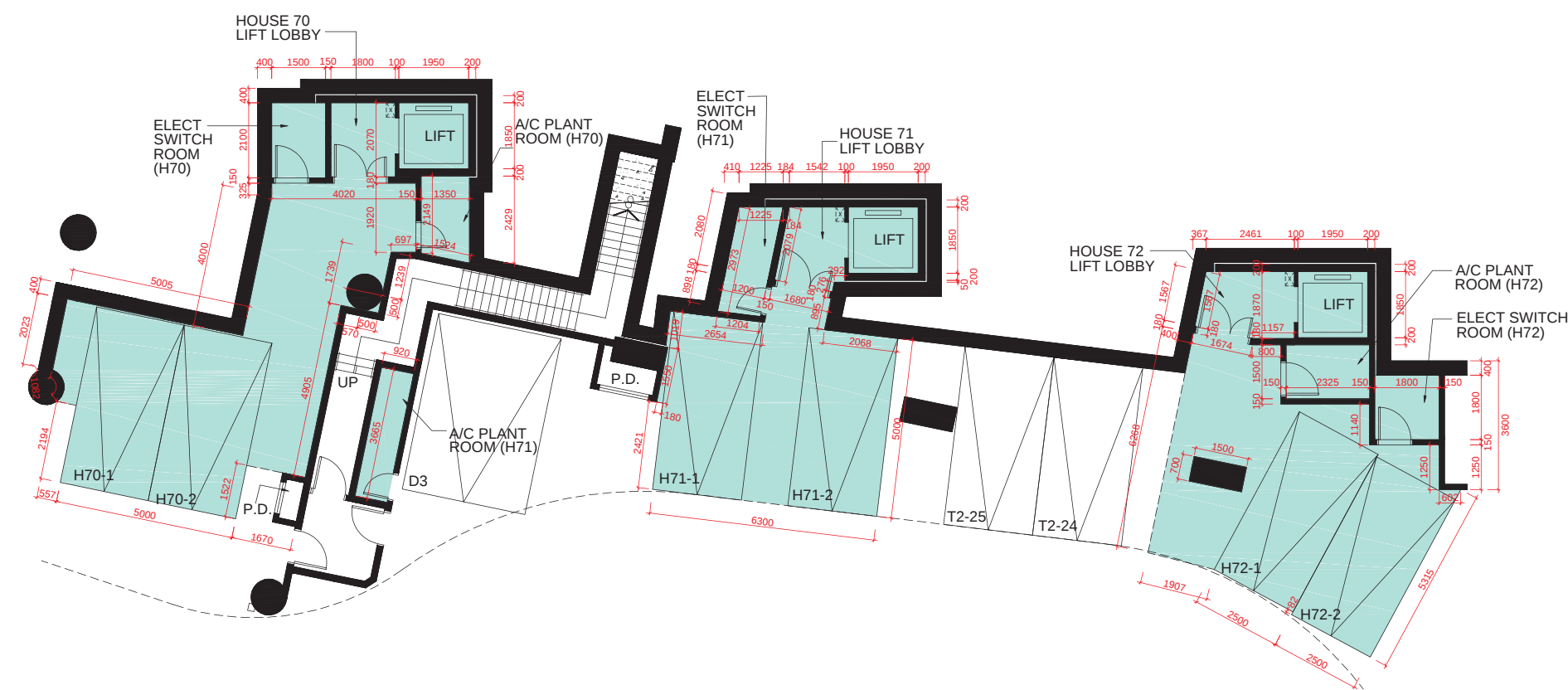
B/F PLAN 地庫層平面圖
