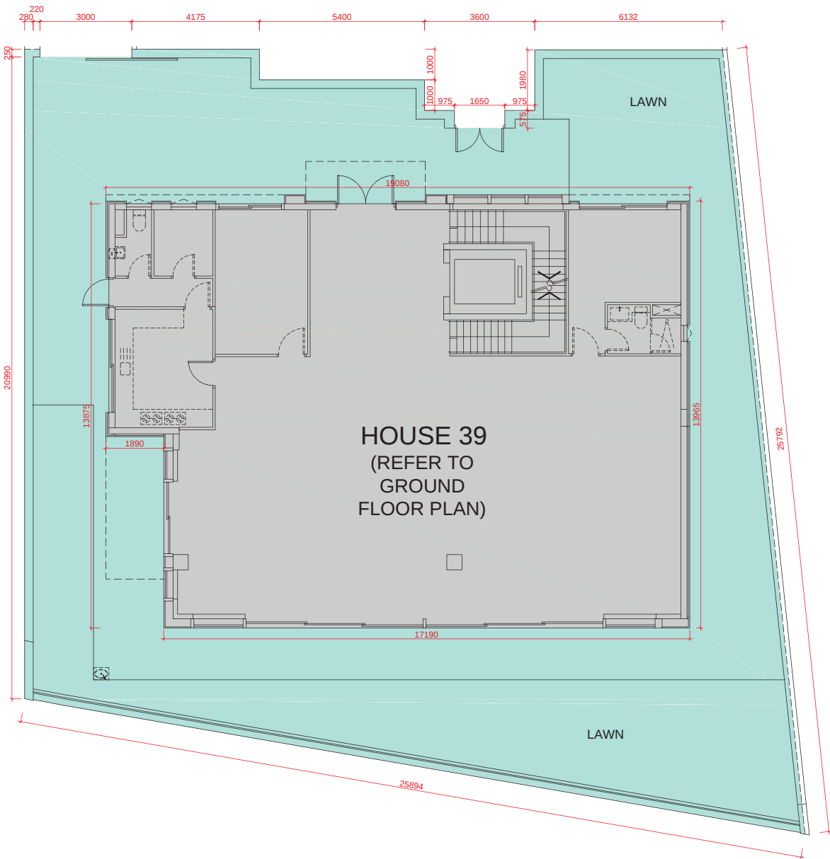
G/F PLAN (FOR GARDEN) 地面層平面圖 (花園)
