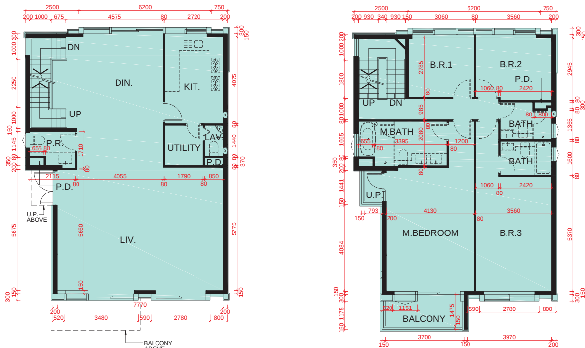
G/F PLAN 地面層平面圖
