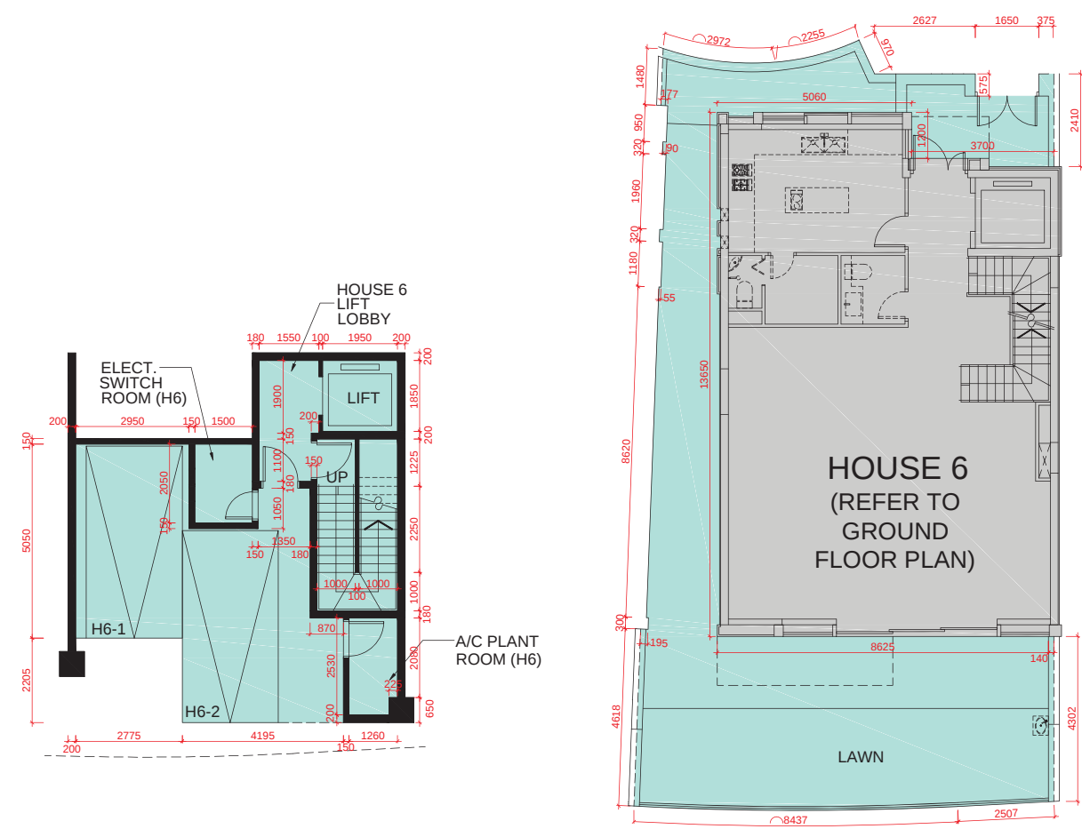
G/F PLAN (FOR GARDEN) 地面層平面圖 (花園)
