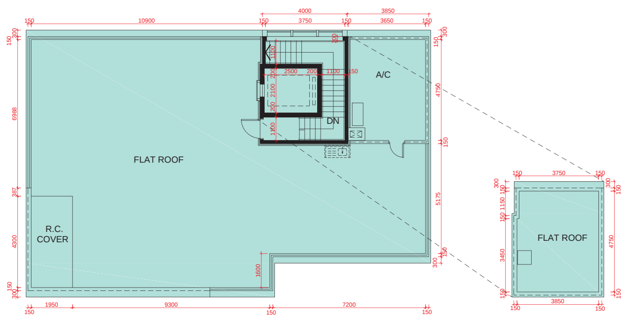
UPPER ROOF PLAN 上層天台平面圖
