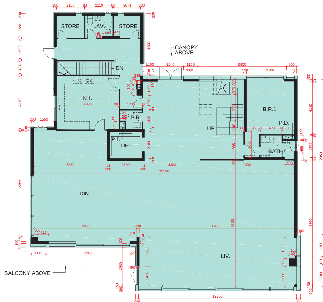
G/F PLAN 地面層平面圖
