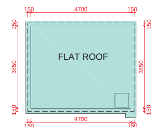
UPPER ROOF PLAN 上層天台平面圖
