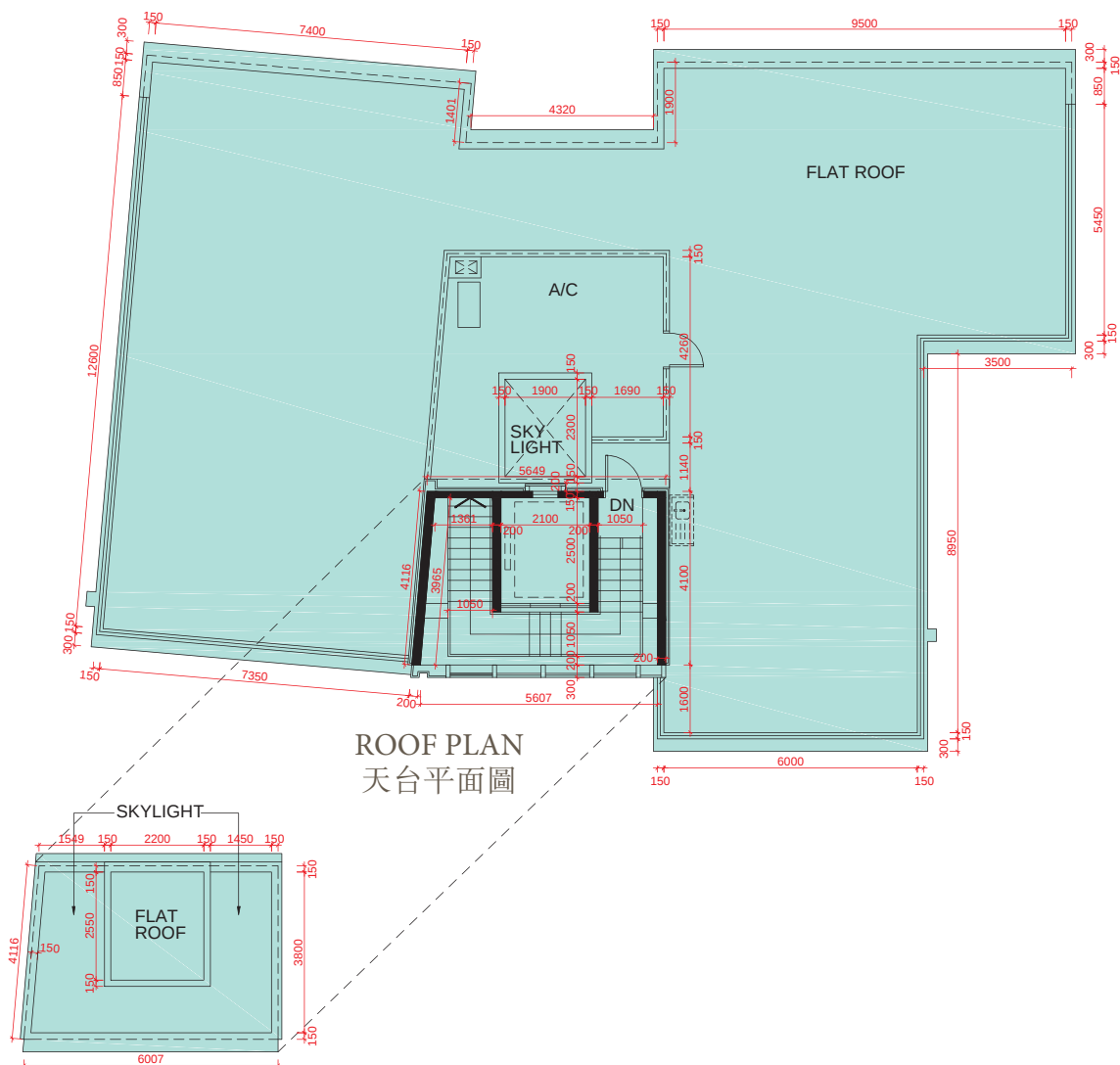
UPPER ROOF PLAN 上層天台平面圖
