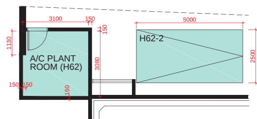
B/F PLAN 地庫層平面圖
