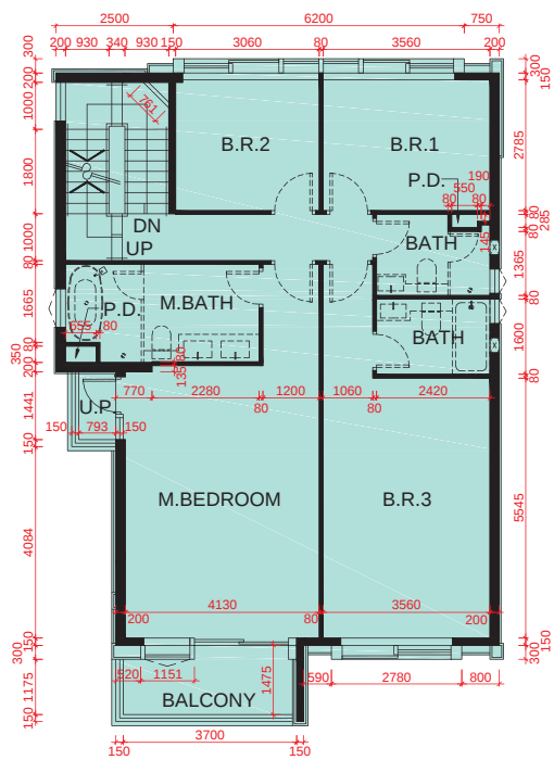
1/F PLAN 1樓平面圖
