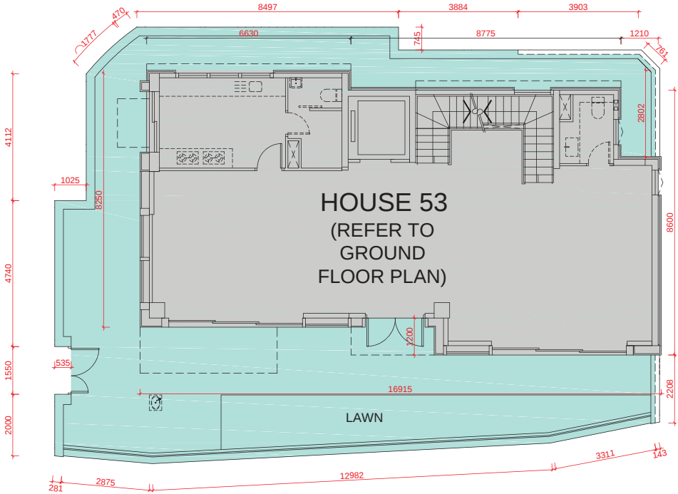
G/F PLAN (FOR GARDEN) 地面層平面圖 (花園)
