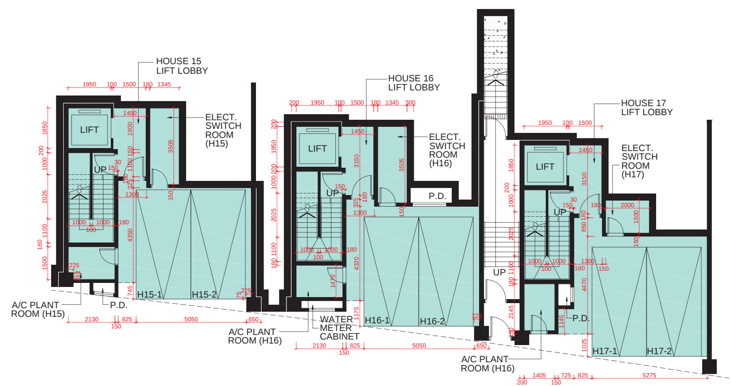
B/F PLAN 地庫層平面圖
