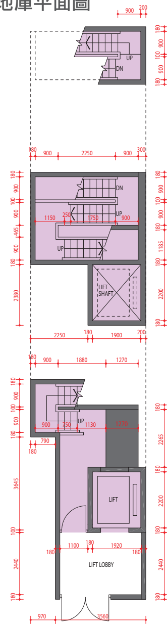
B/F Floor Plan 地庫平面圖
