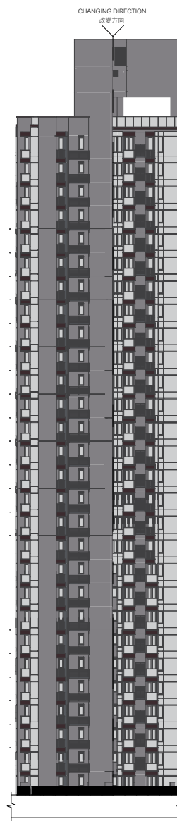
Elevation Plan D 立面圖 D
