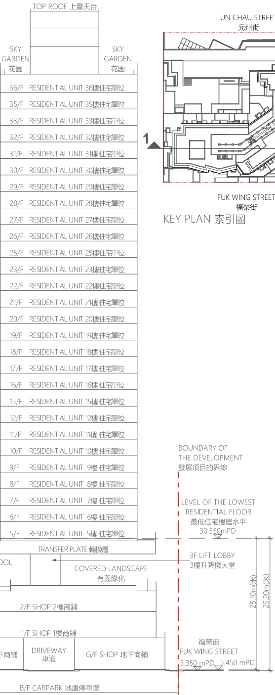
CROSS-SECTION PLAN 2 橫截面圖 2
