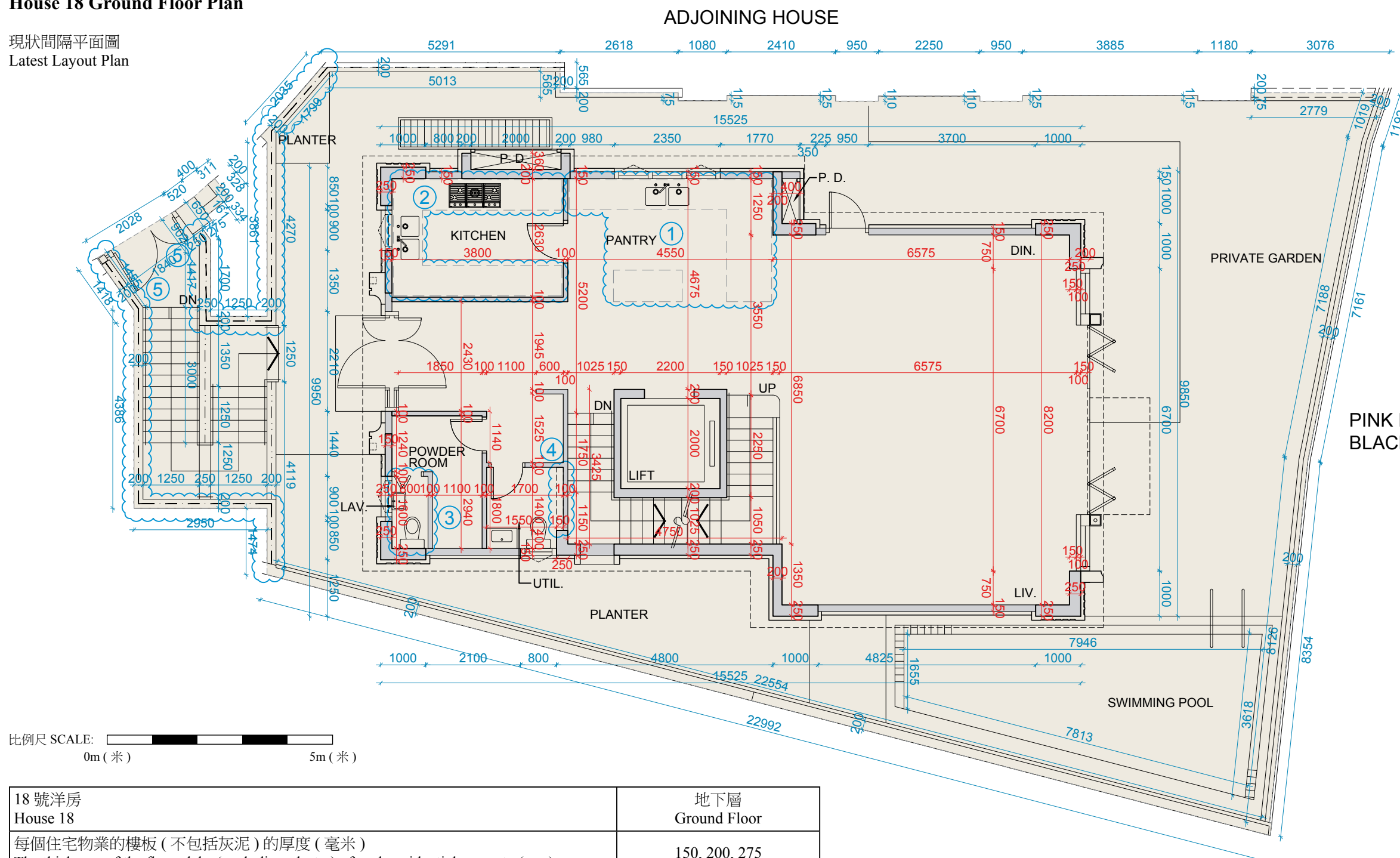
18 號洋房地下層平面圖 House 18 Ground Floor Plan
