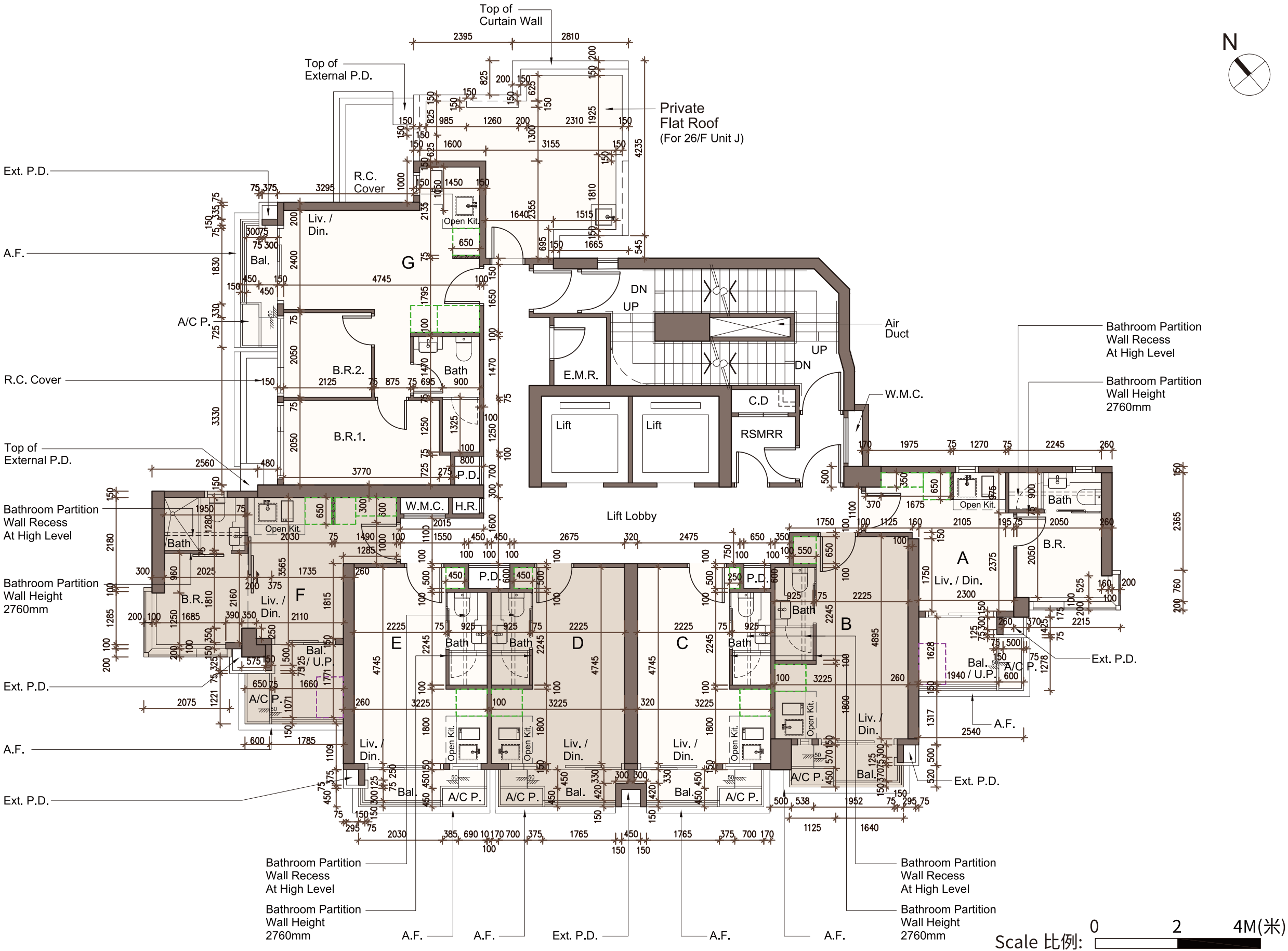
27/F Floor Plan 27樓樓面平面圖
