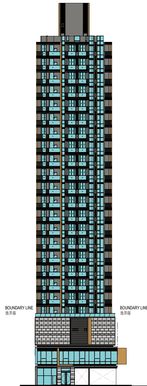
SOUTH EAST ELEVATION 東南立面圖
