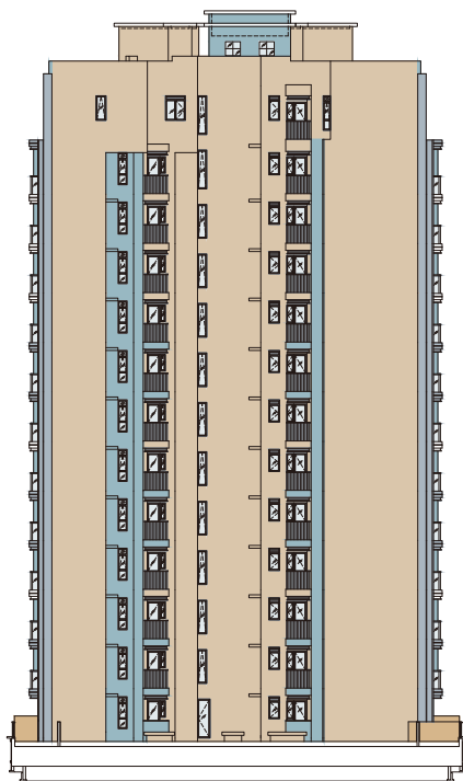
Elevation 1 立面 1
