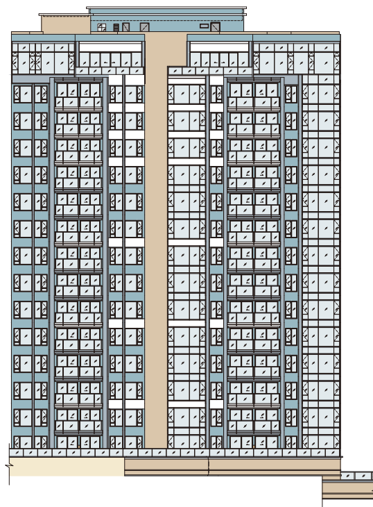
Elevation 2 立面 2
