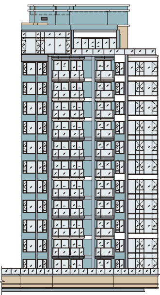
Elevation 3 立面 3
