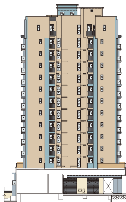
Elevation 4 立面 4
