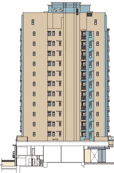
Elevation 4 立面 4
