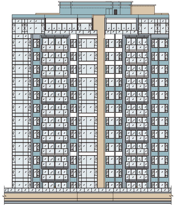
Elevation 4 立面 4
