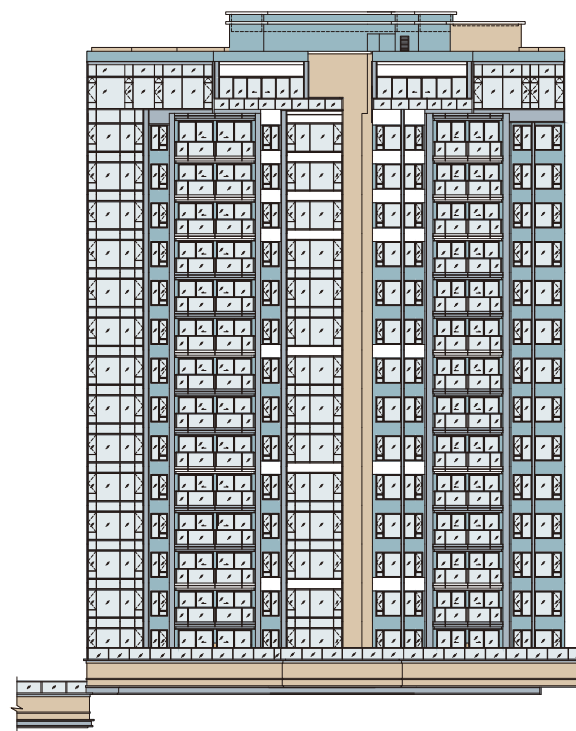
Elevation 4 立面 4
