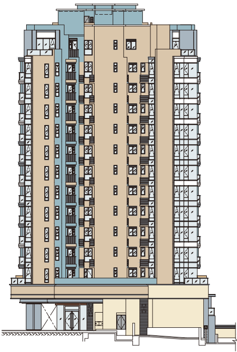
Elevation 2 立面 2
