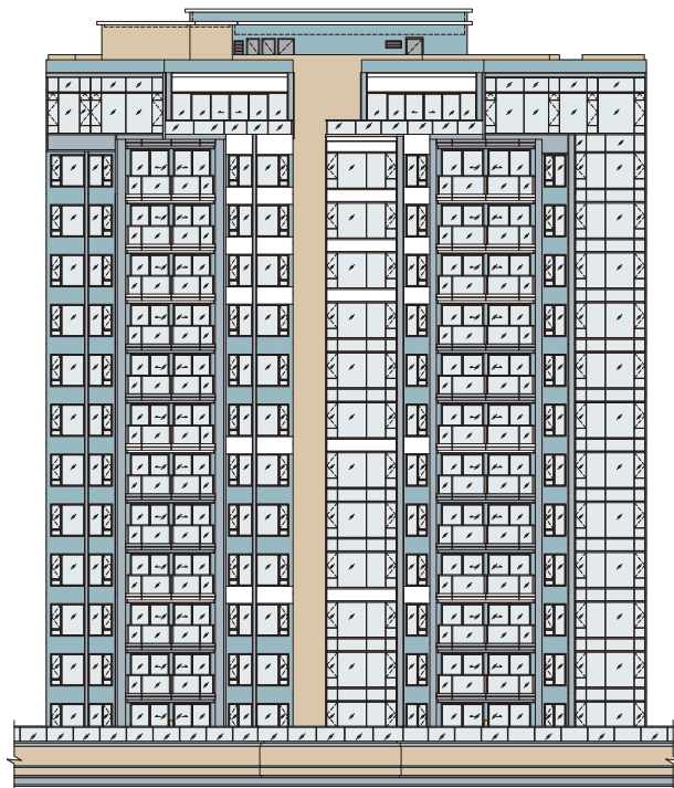
Elevation 2 立面 2
