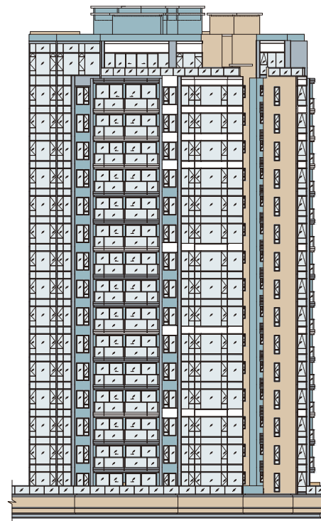
Elevation 4 立面 4
