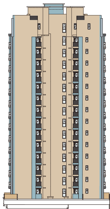
Elevation 3 立面 3
