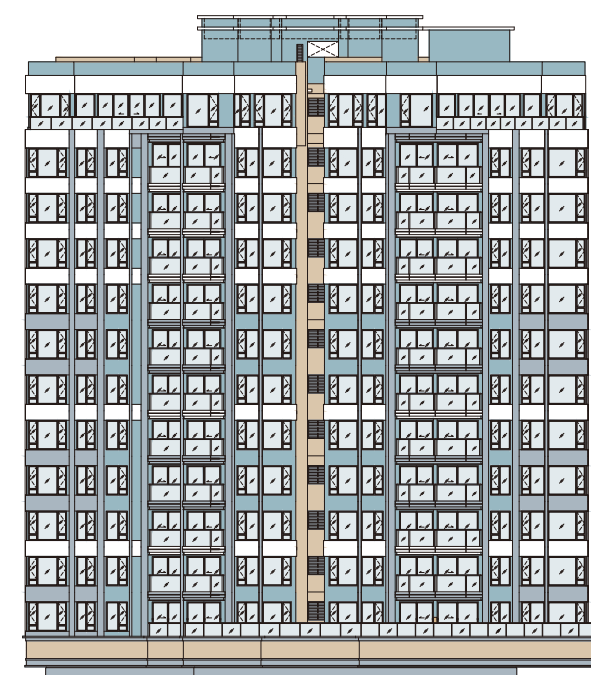
Elevation 4 立面 4
