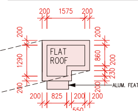
TOP ROOF PART PLAN 天台頂層局部平面圖
