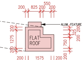
TOP ROOF PART PLAN 天台頂層局部平面圖
