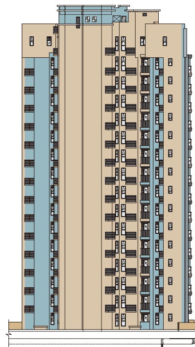
Elevation 2 立面圖 2
