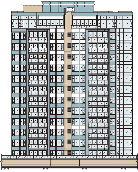
Elevation 4 立面圖 4
