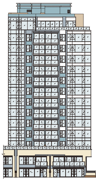
Elevation 1 立面圖 1
