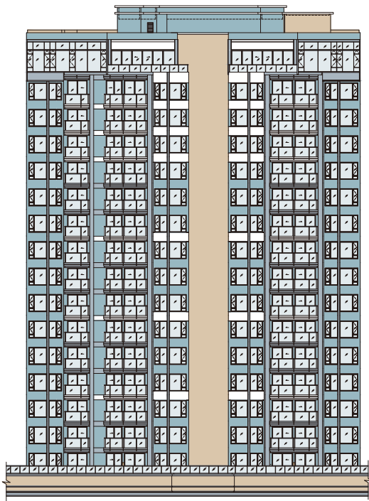
Elevation 2 立面圖 2
