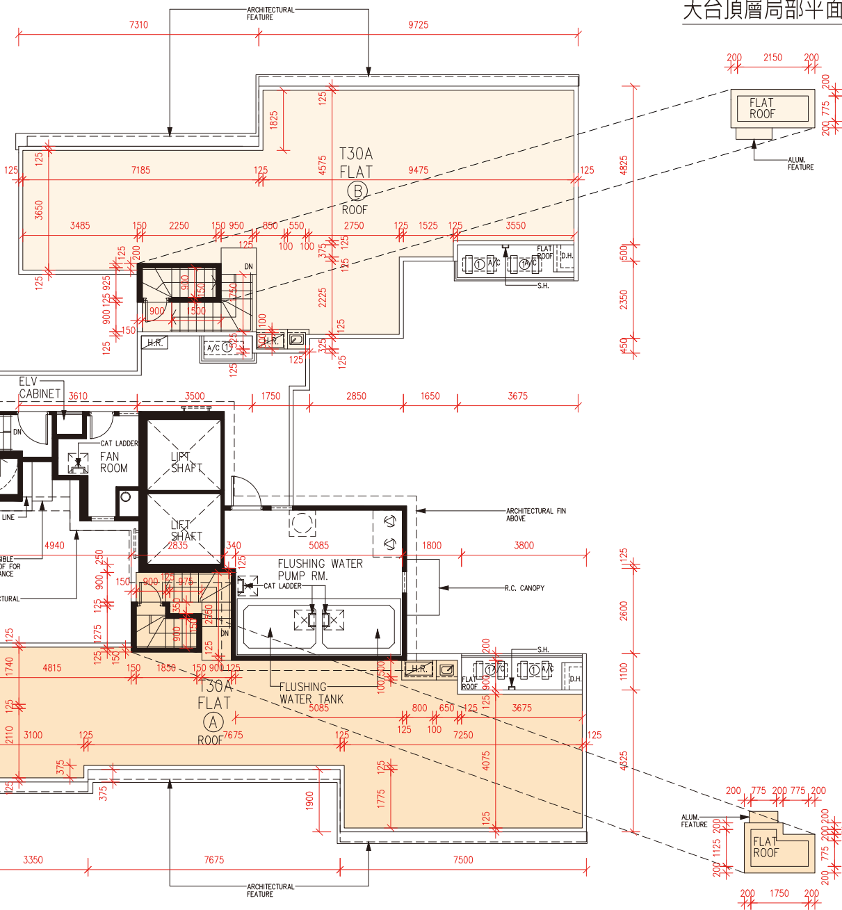
TOP ROOF PART PLAN 天台頂層局部平面圖
