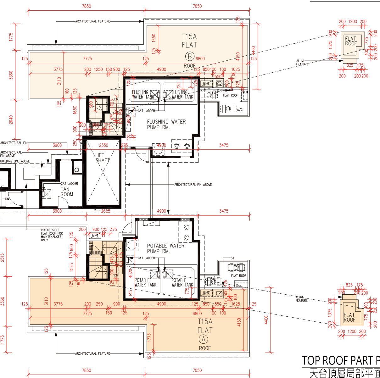
TOP ROOF PART PLAN 天台頂層局部平面圖
