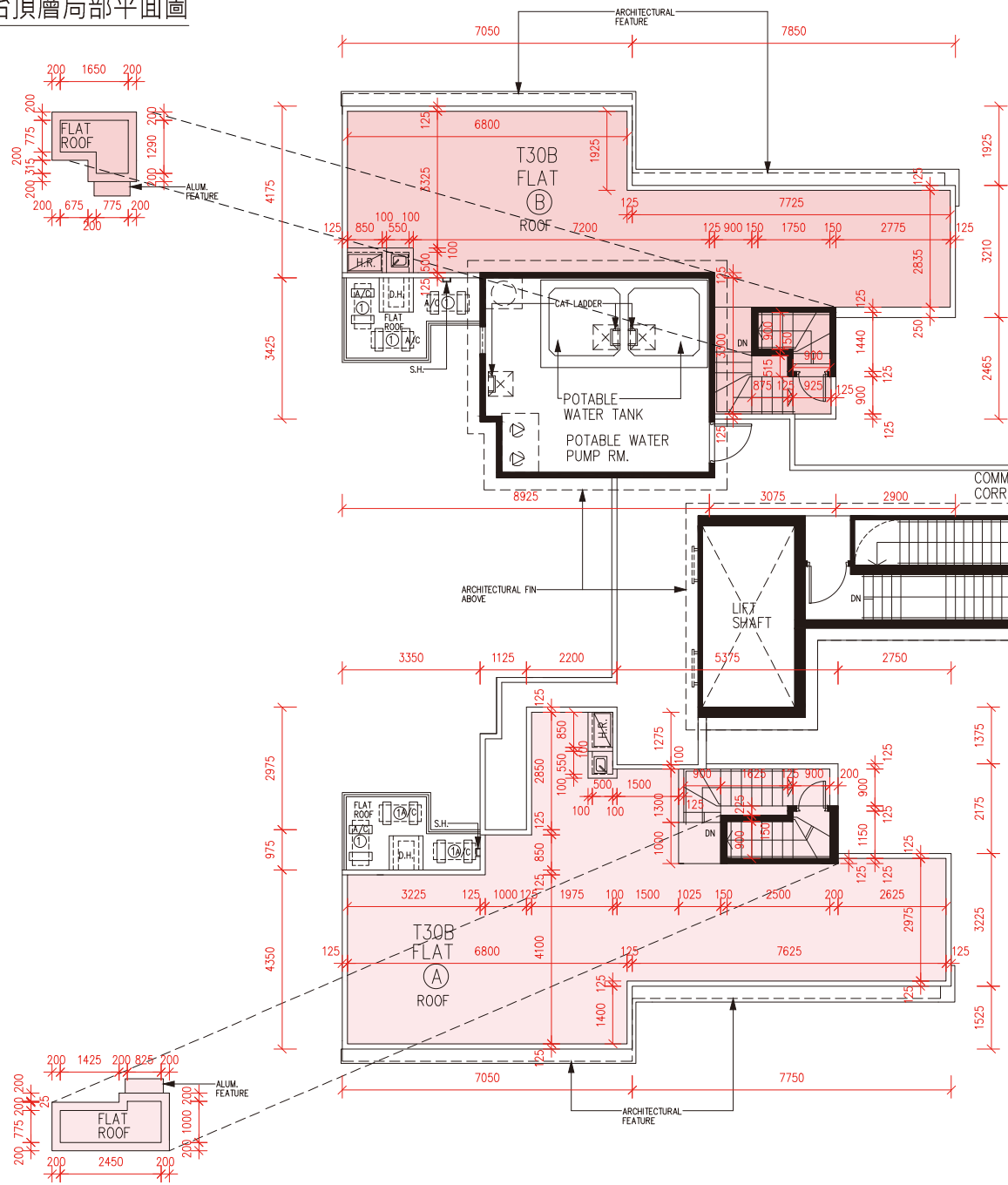
TOP ROOF PART PLAN 天台頂層局部平面圖
