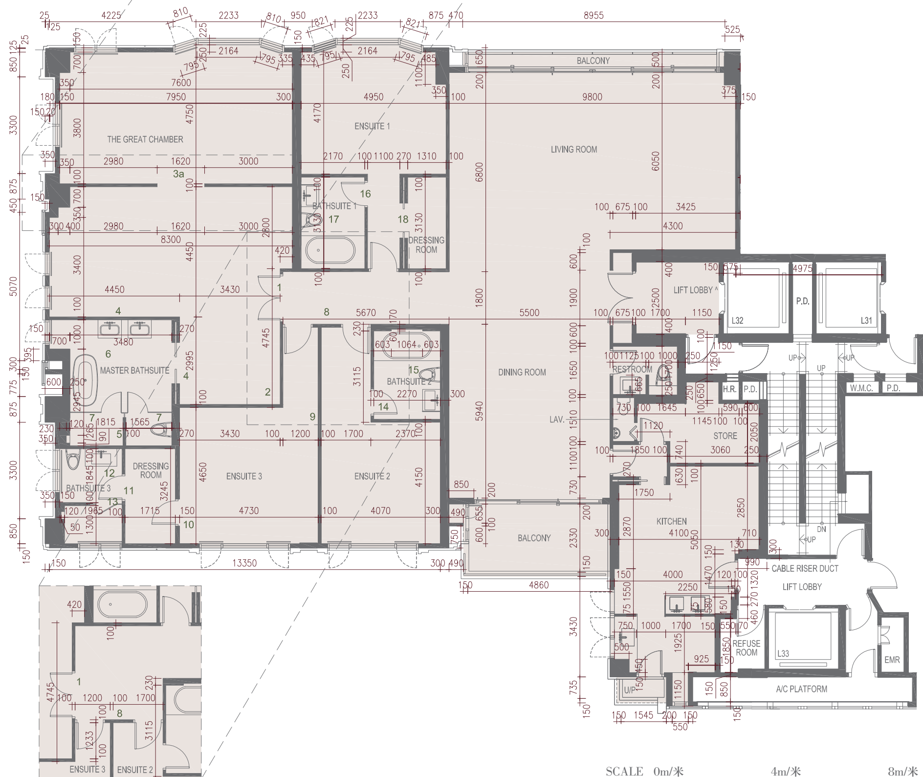
PART PLAN SHOWING LATEST LAYOUT OF 9/F 九樓現狀間隔部份平面圖
