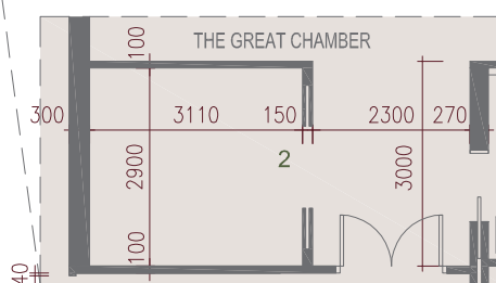
PART PLAN SHOWING LATEST LAYOUT OF 8/F 八樓現狀間隔 部份平面圖
