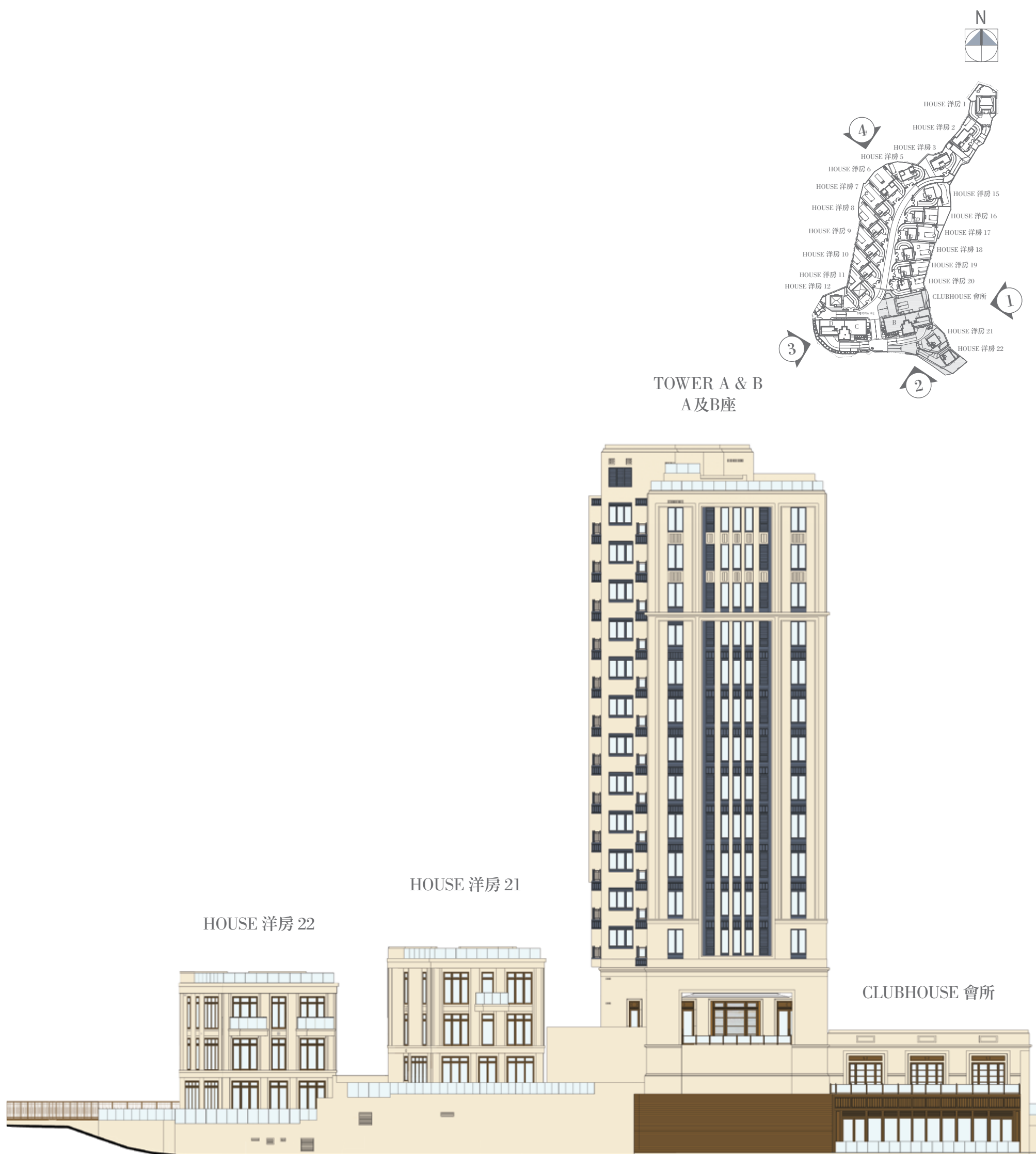
Elevation 1 立面圖一
