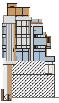
ELEVATION 4 立面圖4
