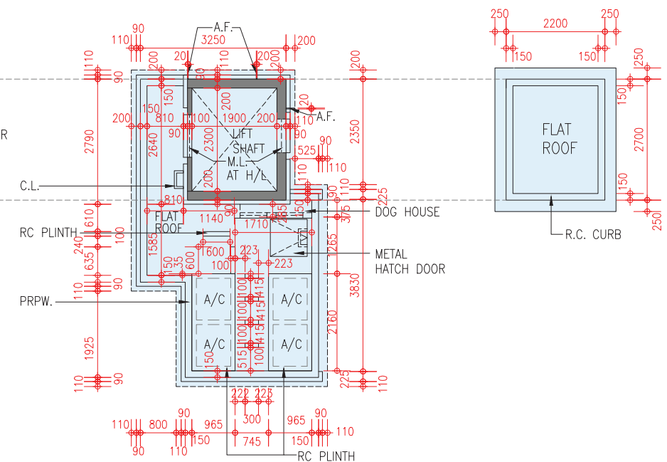
Upper Roof Floor Plan 上層天台樓面平面圖
