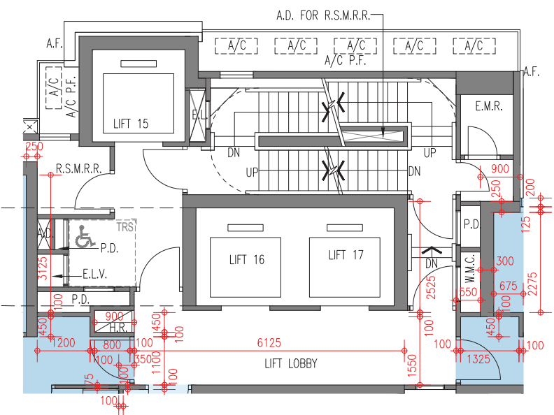
Part plan of Tower 6 - 37/F 第6座37樓之部份平面圖
