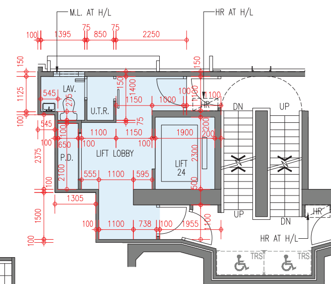
2/F Floor Plan 2樓樓面平面圖
