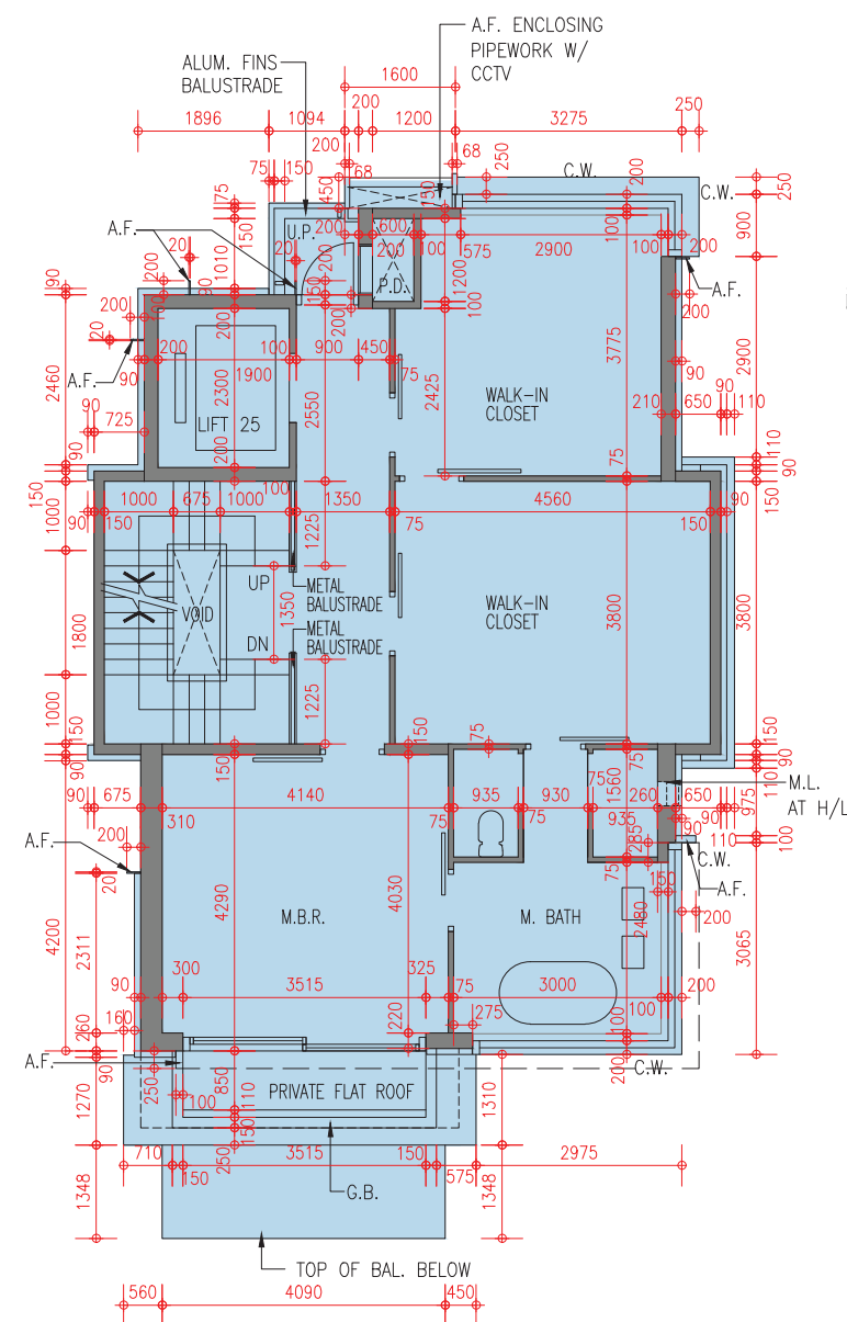
6樓樓面平面圖
