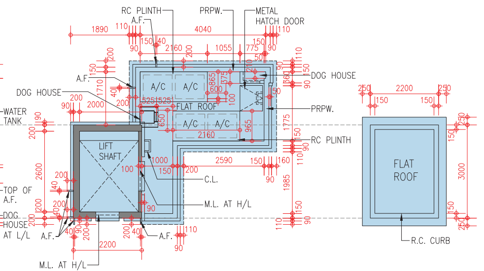
Upper Roof Floor Plan 上層天台樓面平面圖
