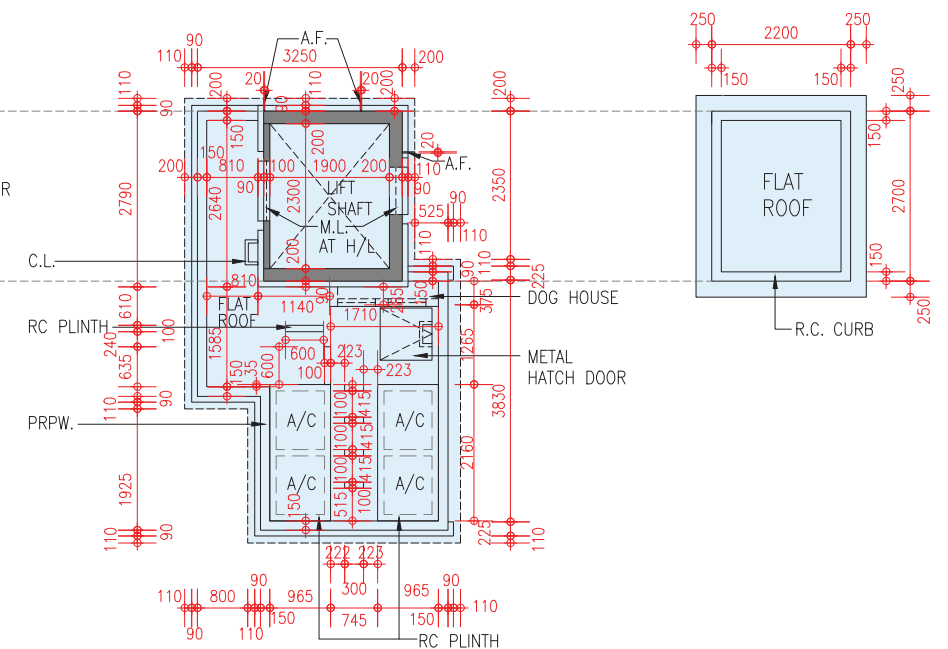
Upper Roof Floor Plan 上層天台樓面平面圖
