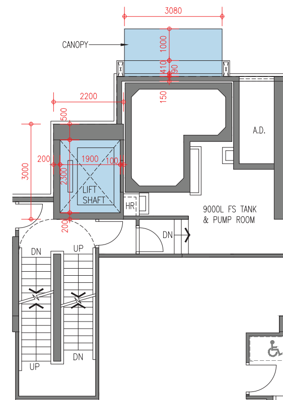
1/F Floor Plan 1樓樓面平面圖
