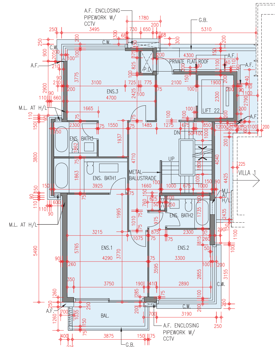
5/F Floor Plan 5樓樓面平面圖
