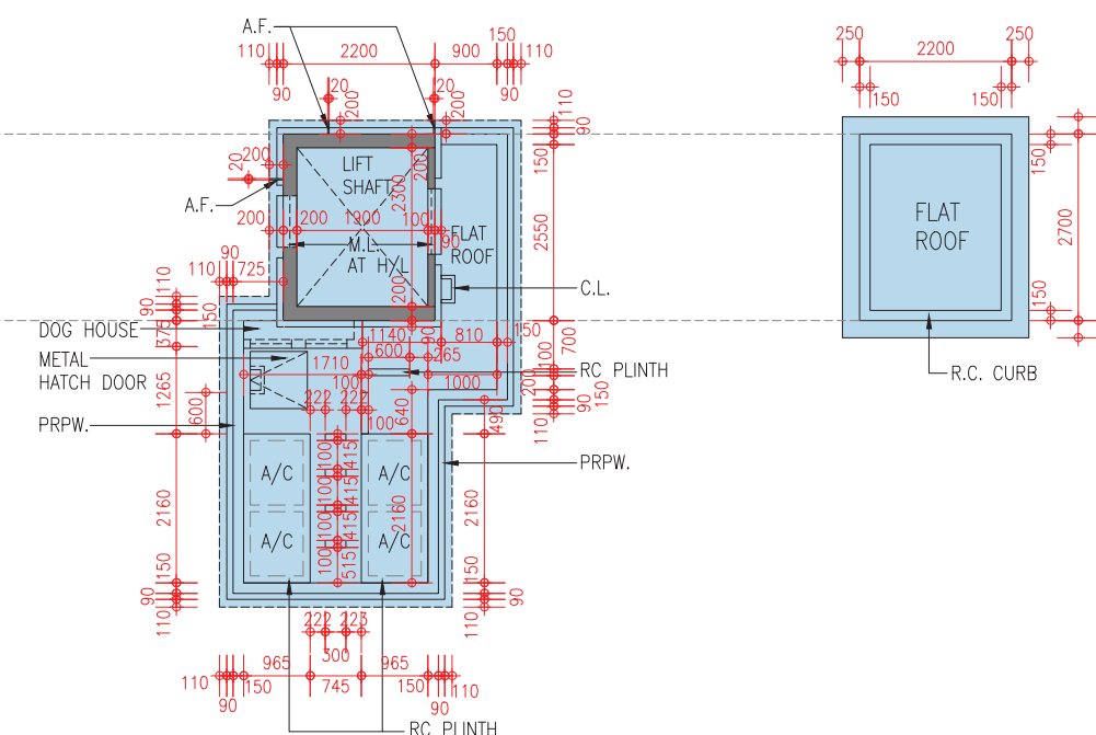
上層天台樓面平面圖
