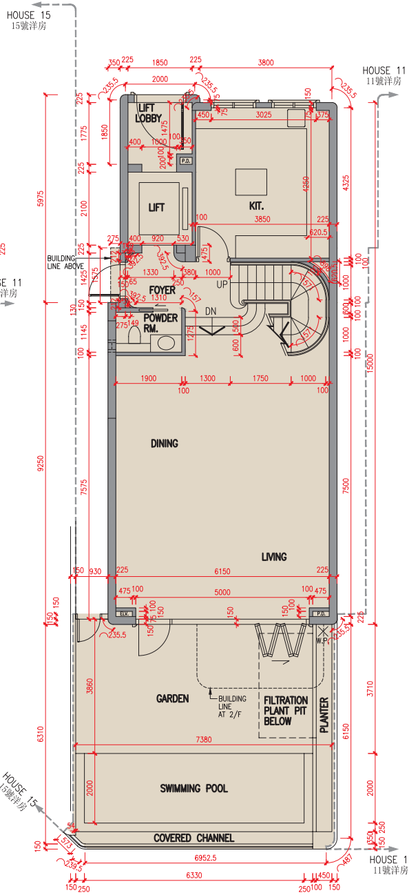
地下平面圖 G/F Plan
