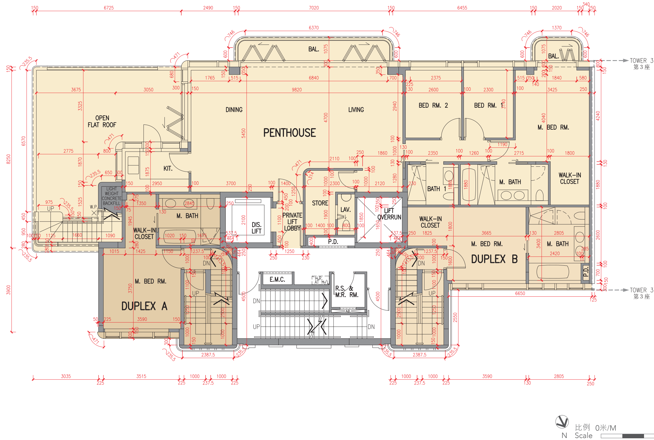
6樓平面圖 6/F Plan
