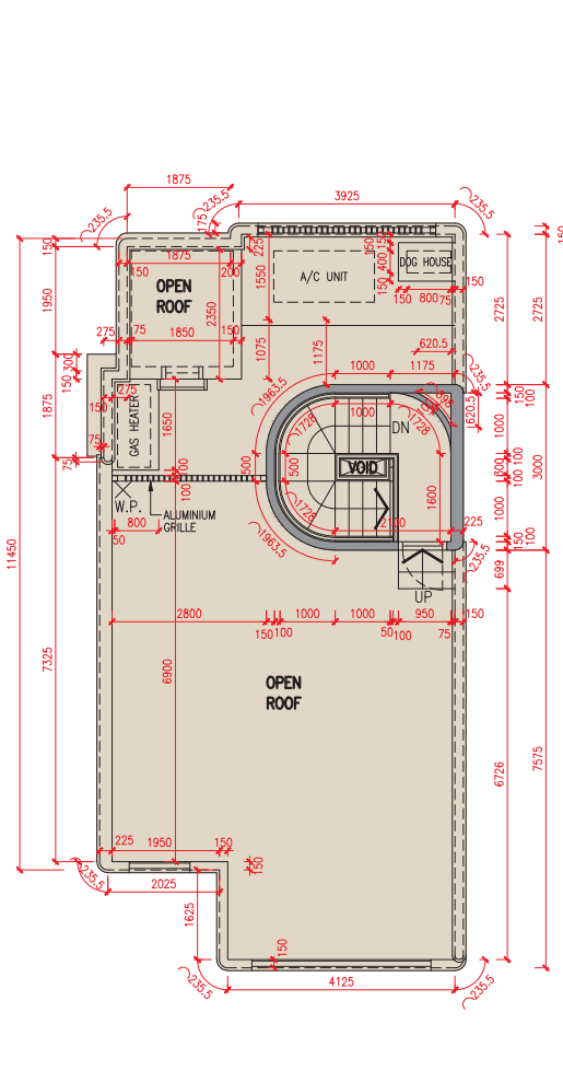
天台平面圖 Roof Plan
