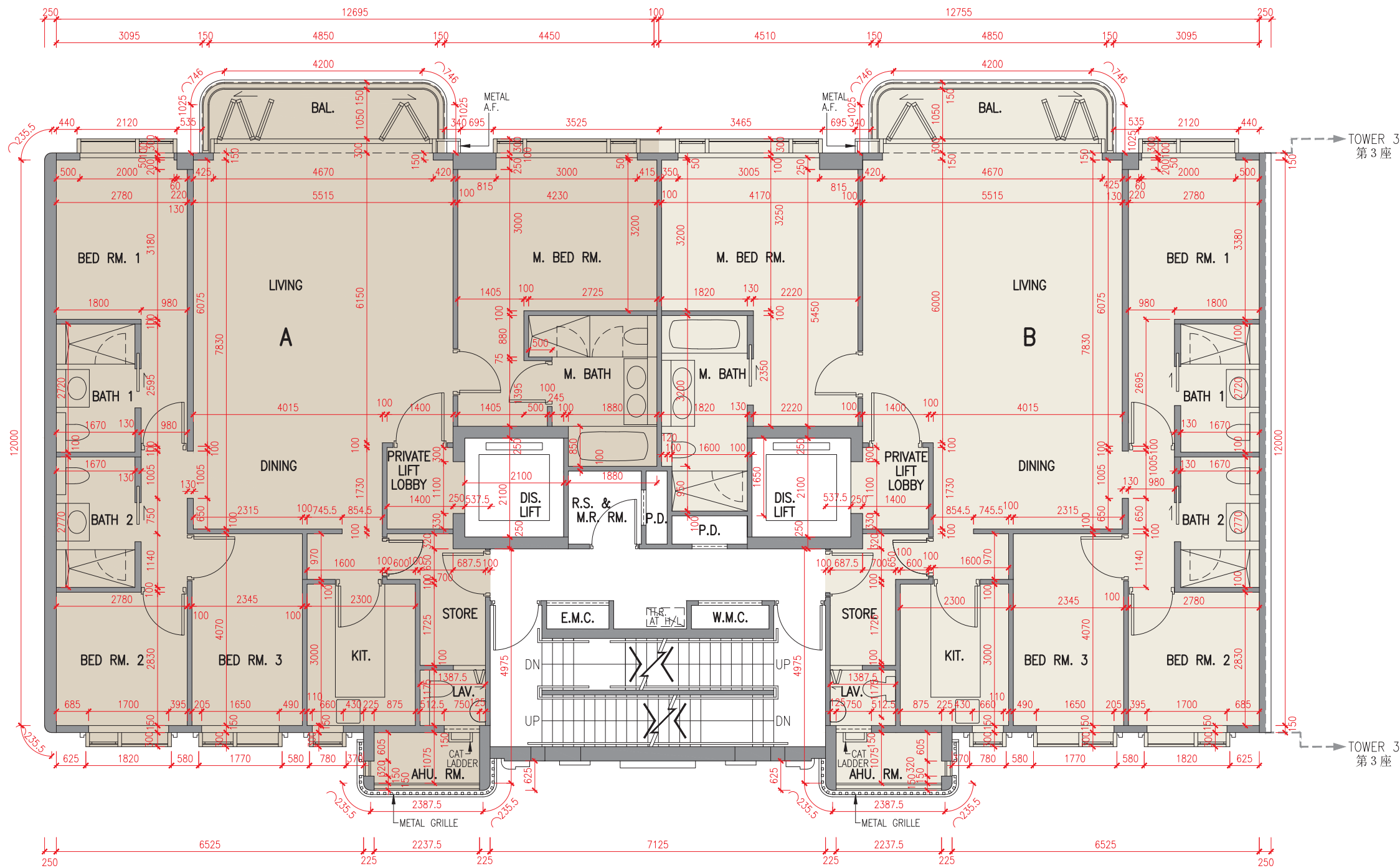
3樓平面圖 3/F Plan
