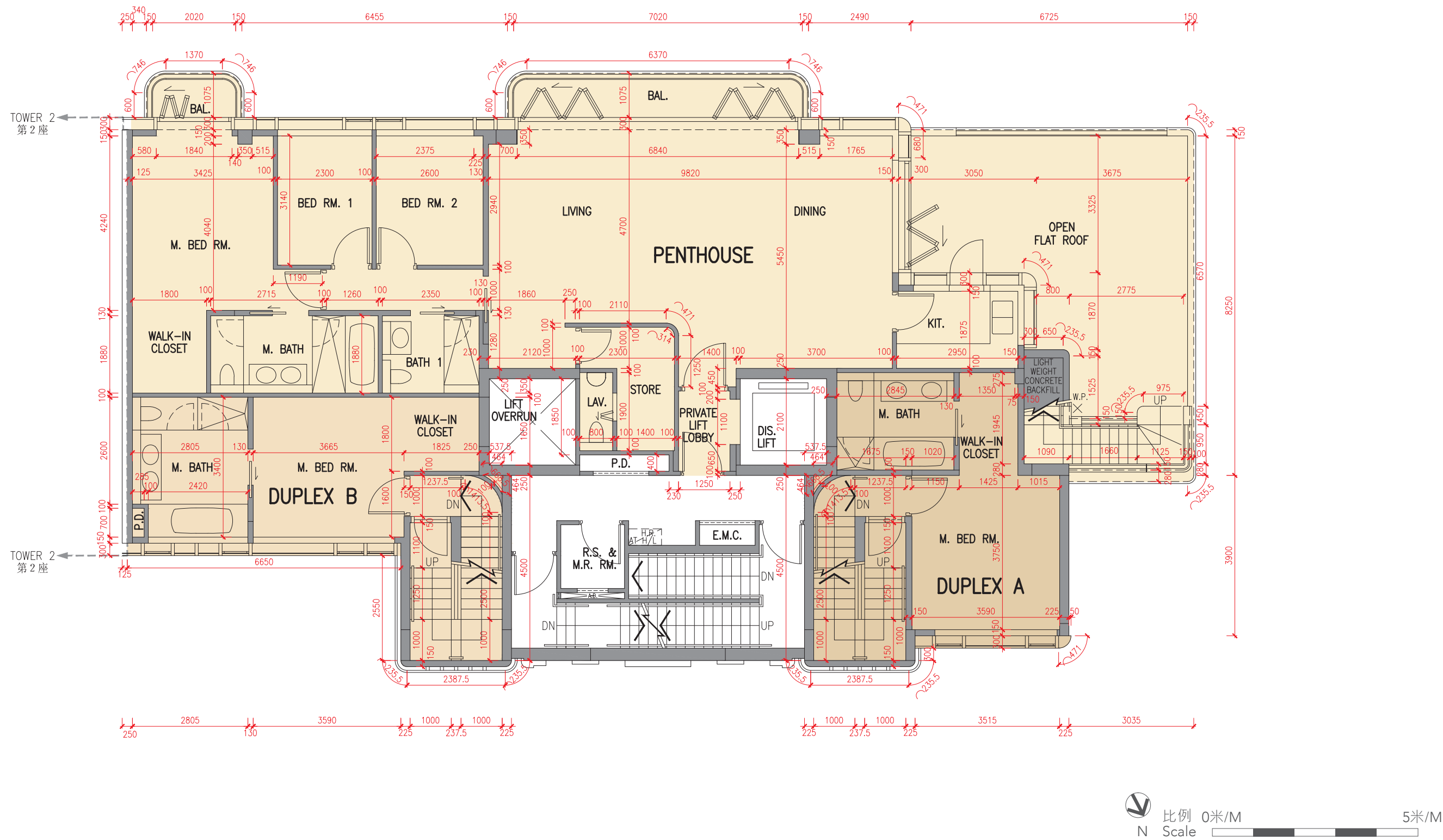
6樓平面圖 6/F Plan
