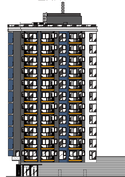
Elevation 5 立面圖5
