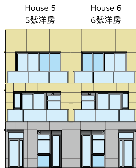
Elevation Plan 1 立面圖 1
