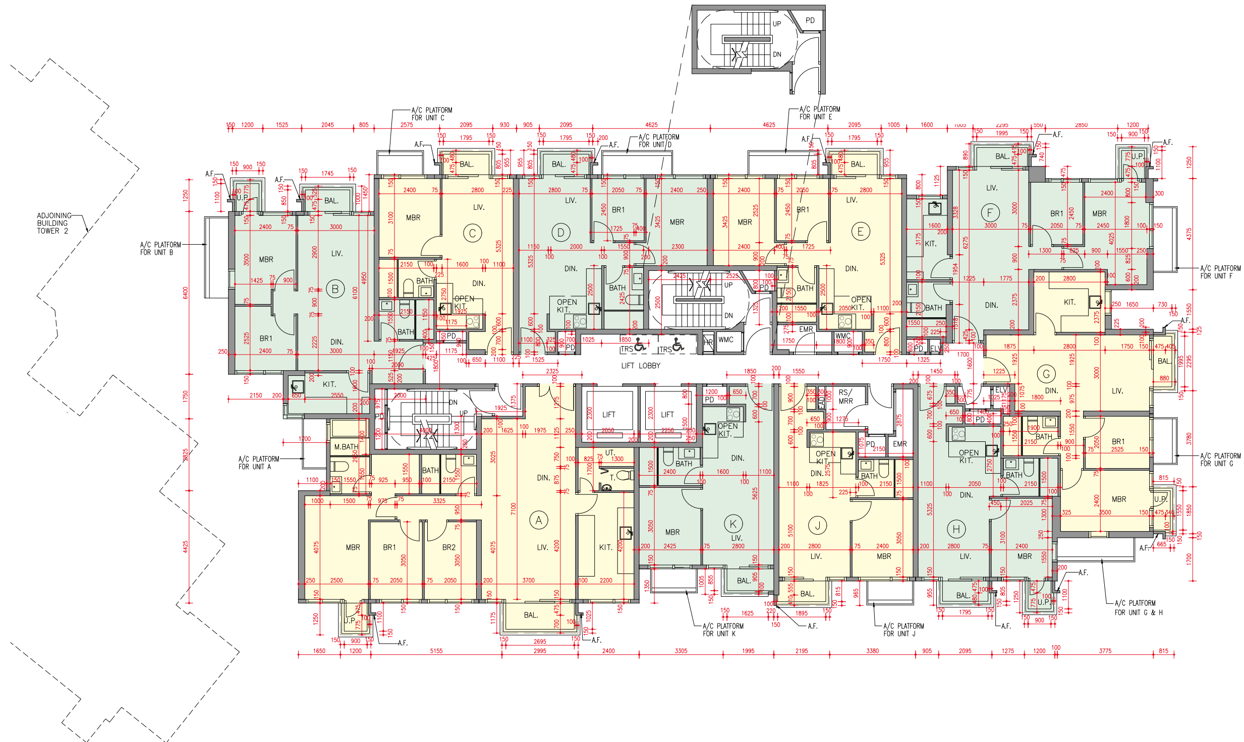
Tower 1 20/F Part Plan 第1座20樓局部平面圖
