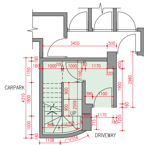
B1/F Floor Plan 地庫一樓樓面平面圖
