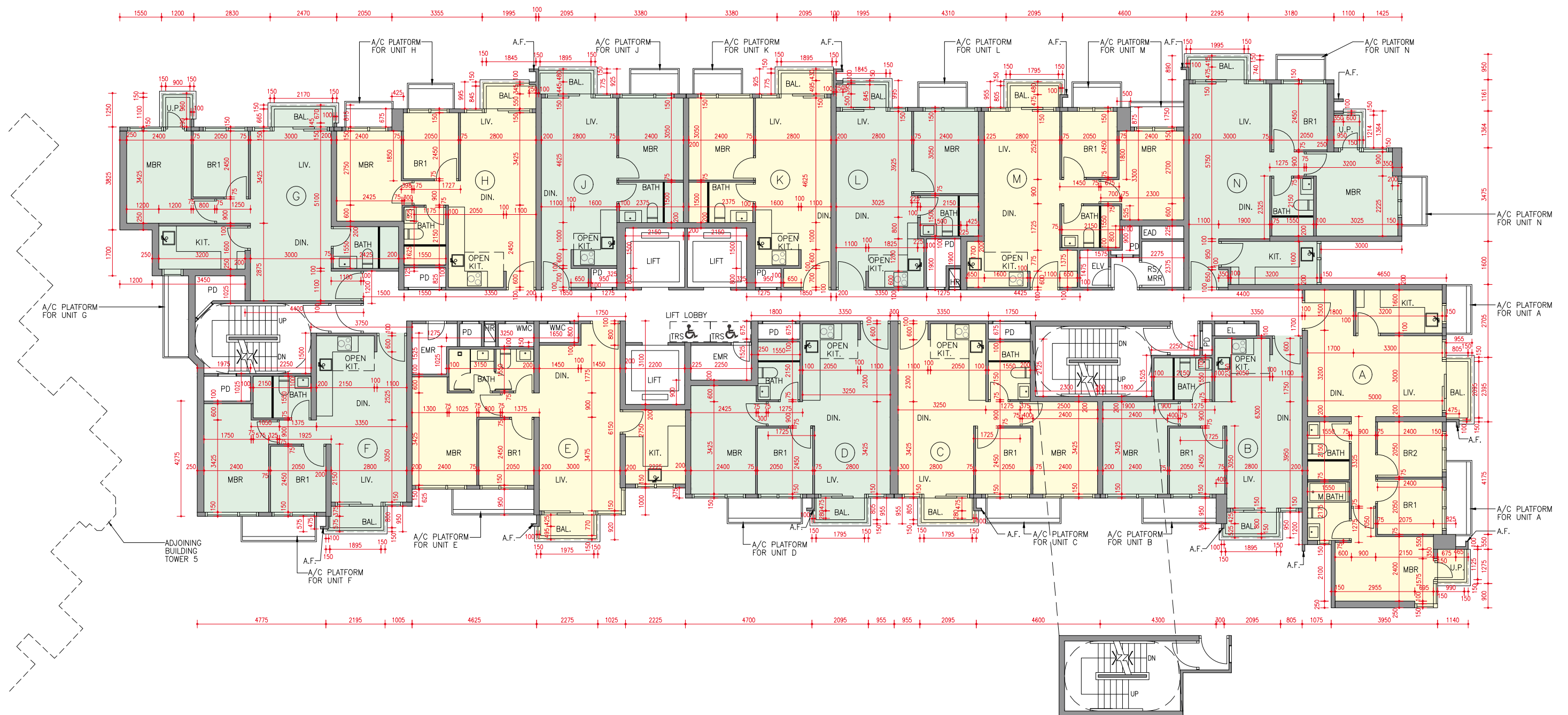
Tower 3 20/F Part Plan 第3座20樓局部平面圖
