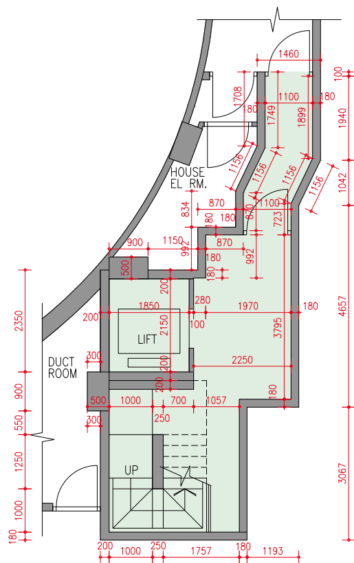
B1/F Floor Plan 地庫一樓樓面平面圖
