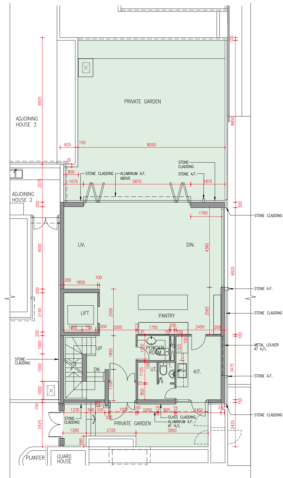
G/F Floor Plan 地下樓面平面圖
