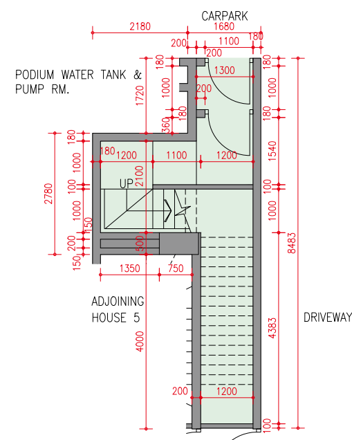
B1/F Floor Plan 地庫一樓樓面平面圖
