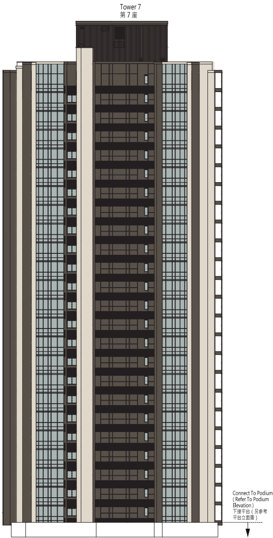
立面圖 C3 Elevation C3
