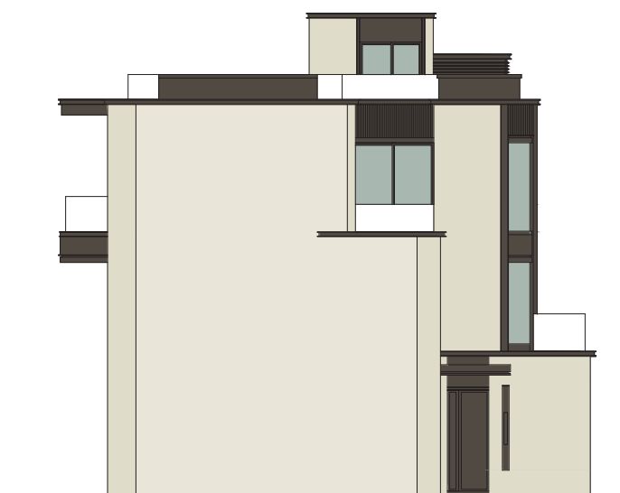
立面圖 C1 (適用於 C5 洋房) Elevation C1 (For House C5)
