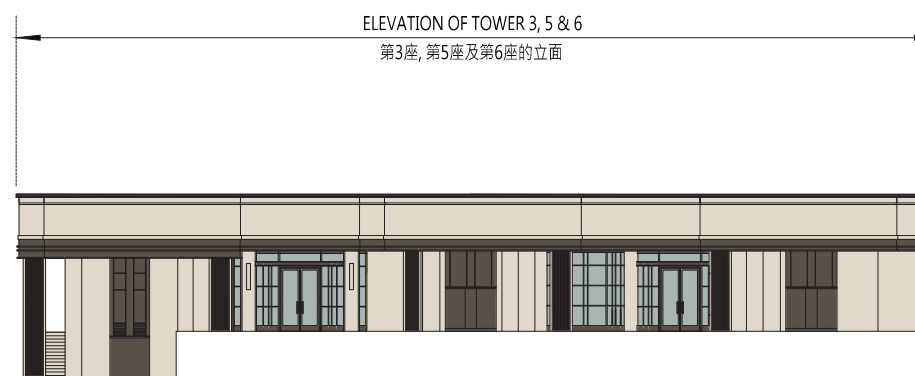
平台立面圖 B1 Podium Elevation B1
