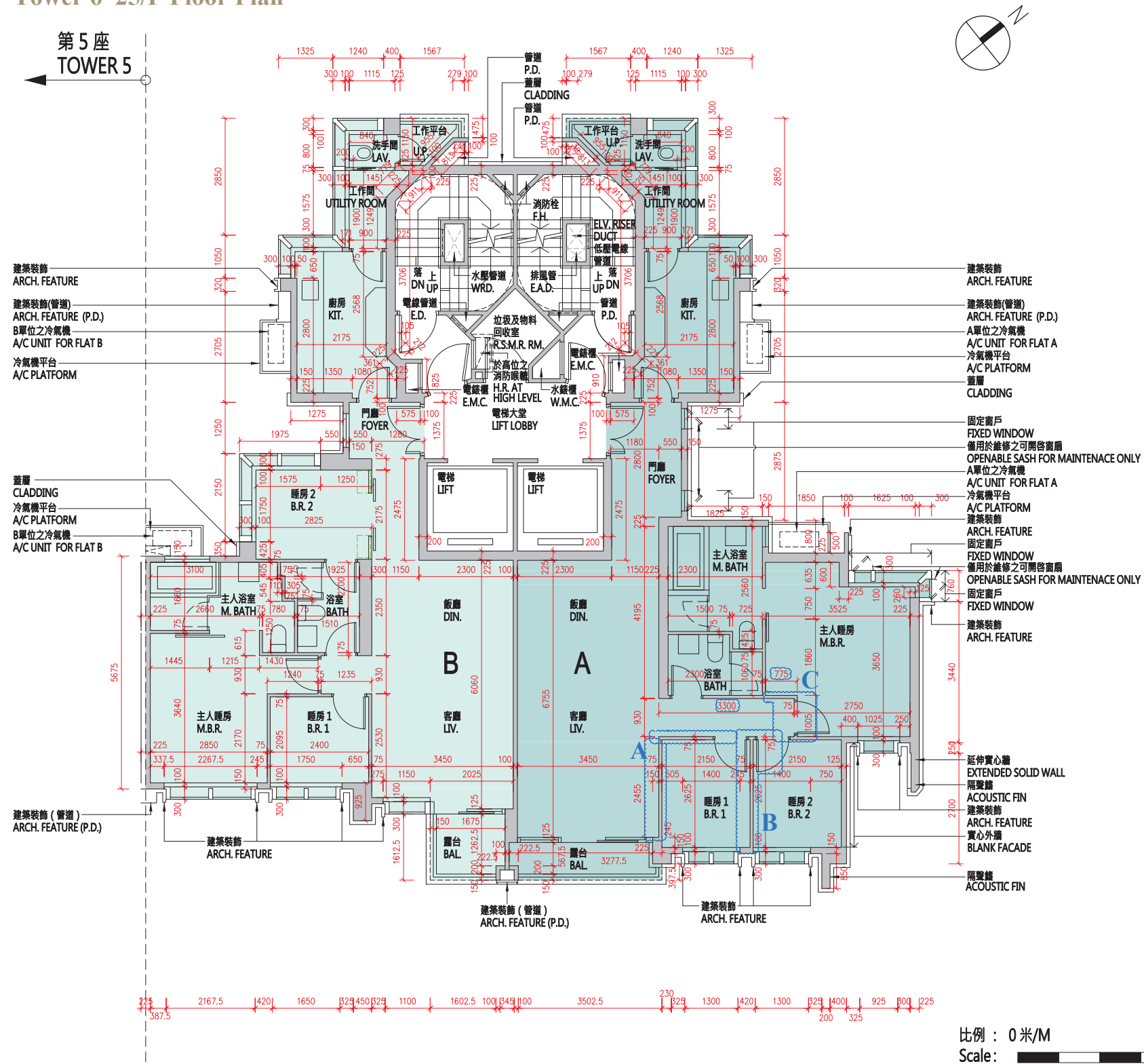
第6座 25樓平面圖 Tower 6 25/F Floor Plan
