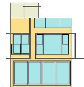
Elevation 2 立面圖 2
