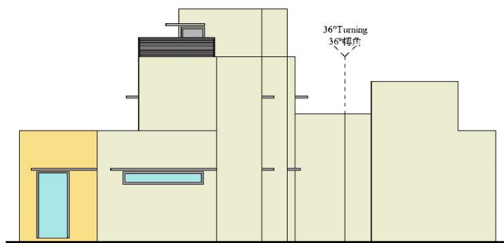
Elevation 3 立面圖 3
