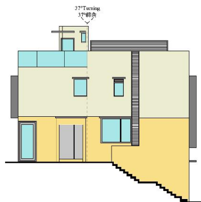
Elevation 3 立面圖 3
