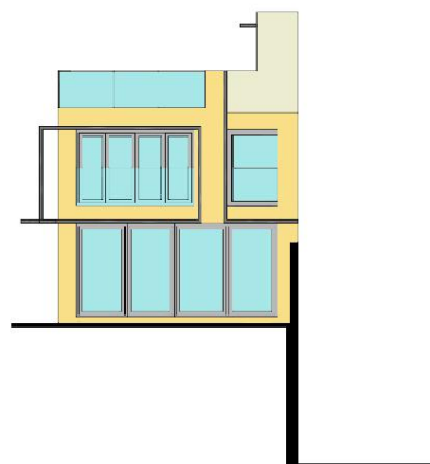
Elevation 1 立面圖 1
