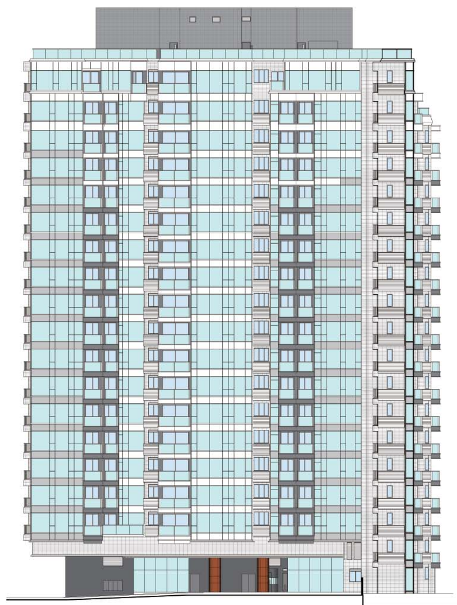
Elevation C1 立面圖 C1
