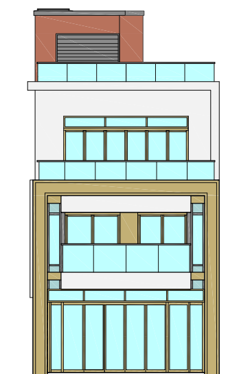
ELEVATION 4 立面圖4
