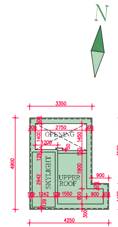
UPPER ROOF PLAN 上層天台平面圖
