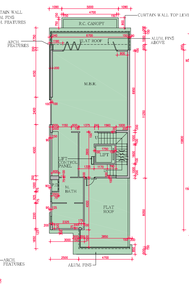
2/F PLAN 2樓平面圖
