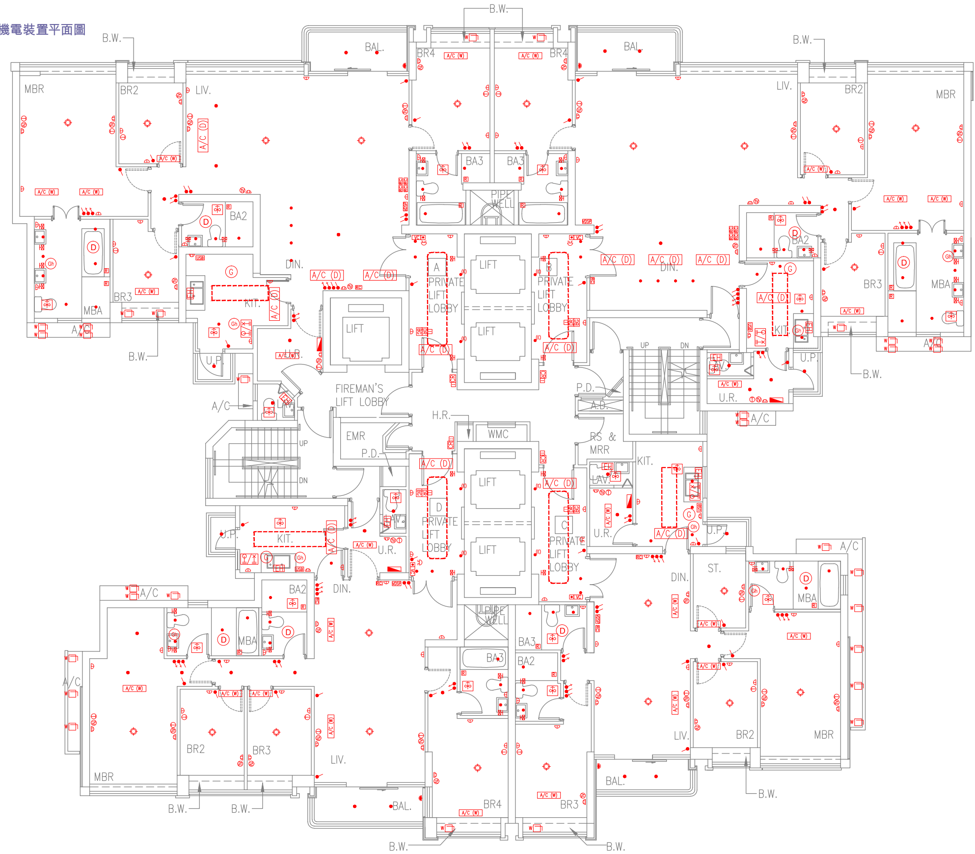
Tower 3 6/F - 12/F, 15/F - 21/F Floor Plan 第3座 6樓至12樓、15樓至21樓面平面圖
