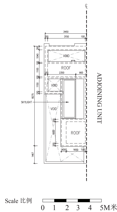
上層天台平面圖 Upper Roof Floor Plan
