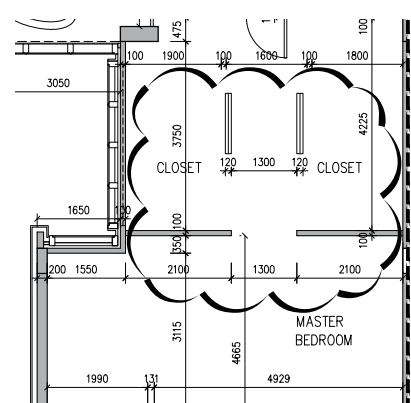
上層天台平面圖 Upper Roof Floor Plan
