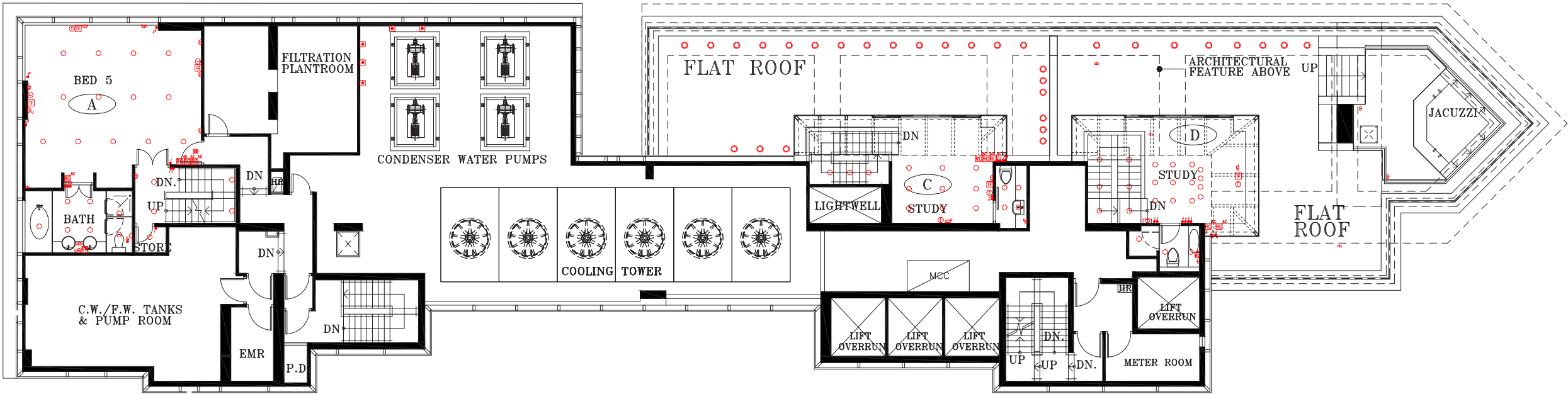
Floor Plan of 92/F. of Zone 1 of Tower 20* 第20座，第1區，92樓平面圖*
