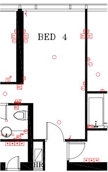
Part Plan of Flat A of 72/F. of Zone 1 of Tower 20* 第20座，第1區，72樓A室部分平面圖*
