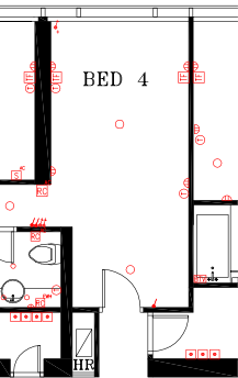
Part Plan of Flat A of 73/F. of Zone 1 of Tower 20* 第20座，第1區，73樓A室部分平面圖*
