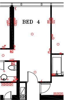
Part Plan of Flat A of 80/F. of Zone 1 of Tower 20* 第20座，第1區，80樓A室部分平面圖*
