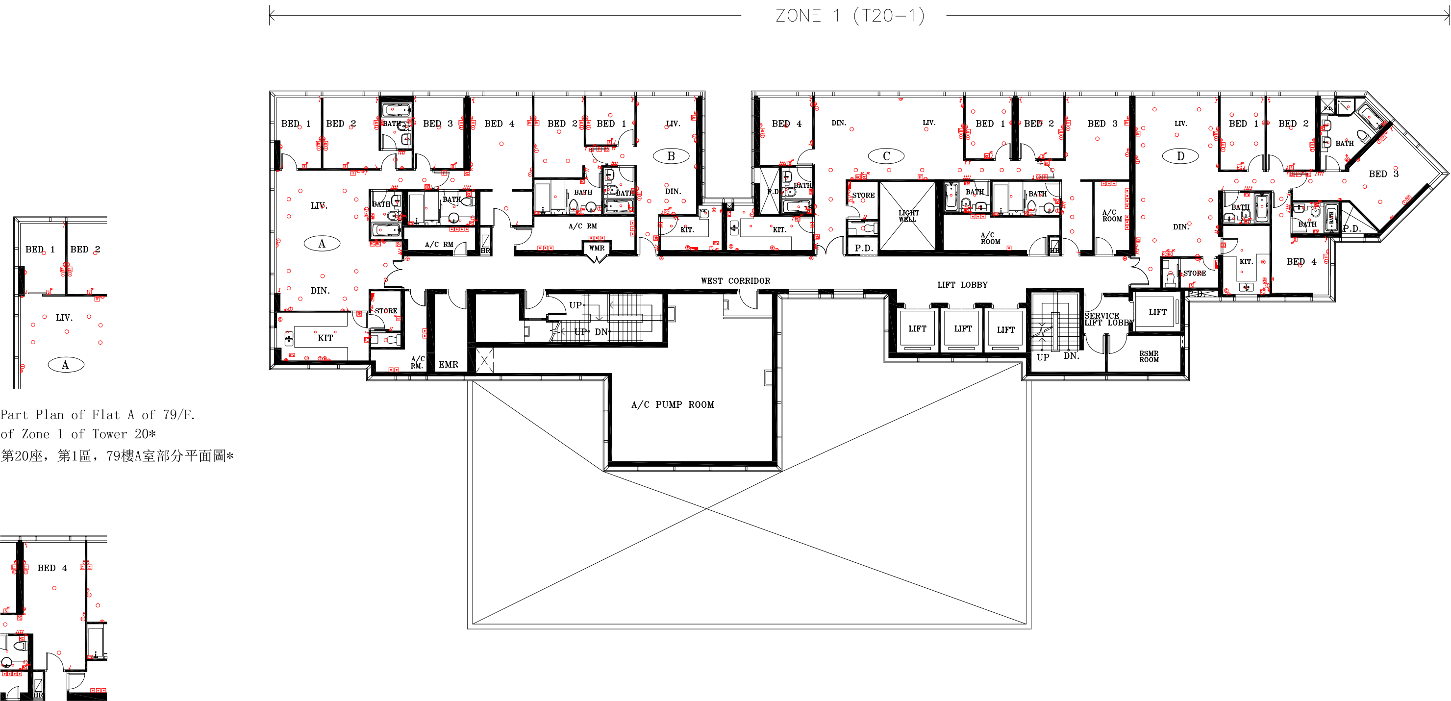
Part Plan of Flat A of 79/F. of Zone 1 of Tower 20* 第20座，第1區，79樓A室部分平面圖*
