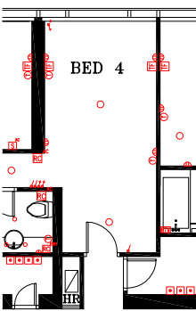
Part Plan of Flat A of 78/F. of Zone 1 of Tower 20* 第20座，第1區，78樓A室部分平面圖*
