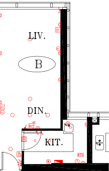
WEST CORRIDOR Part Plan of Flat B of 68/F. of Zone 1 of Tower 20* 第20座，第1區，68樓B室部分平面圖*
