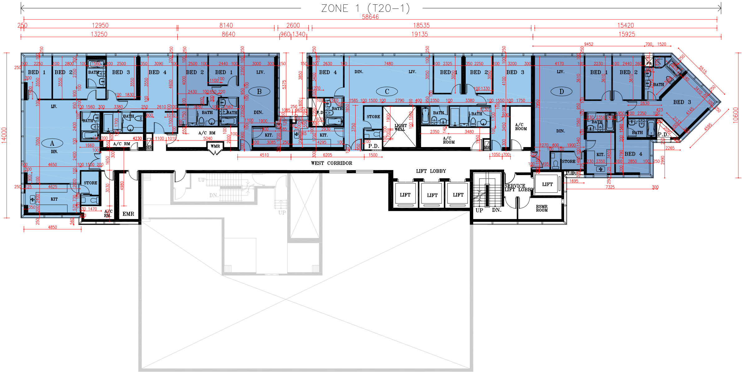
Part Plan of Flat A of 78/F. of Zone 1 of Tower 20* 第20座，第1區，78樓A室部分平面圖*
