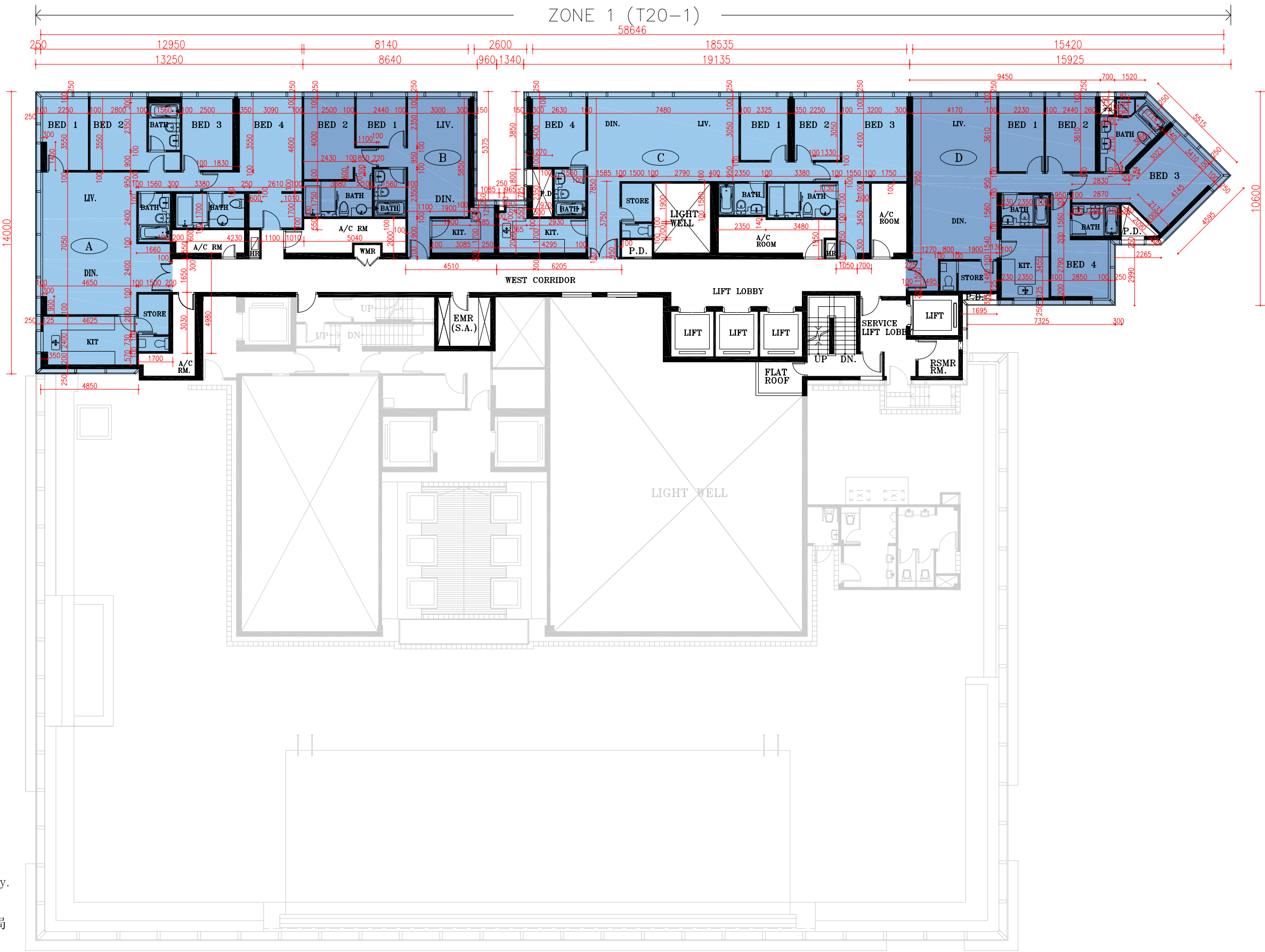
Part Plan of Flat A of 76/F. of Zone 1 of Tower 20* 第20座，第1區，76樓A室部分平面圖*
