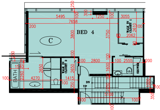
Part Plan of Flat C of 92/F. of Zone 1 of Tower 21* 第21座，第1區，92樓C室部分平面圖*
