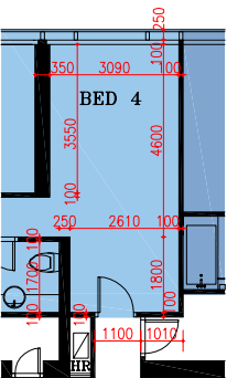
Part Plan of Flat A of 87/F-89/F. of Zone 1 of Tower 20* 第20座，第1區，87樓至89樓A室部分平面圖*
