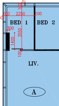
Part Plan of Flat A of 68/F. of Zone 1 of Tower 20* 第20座，第1區，68樓A室部分平面圖*
