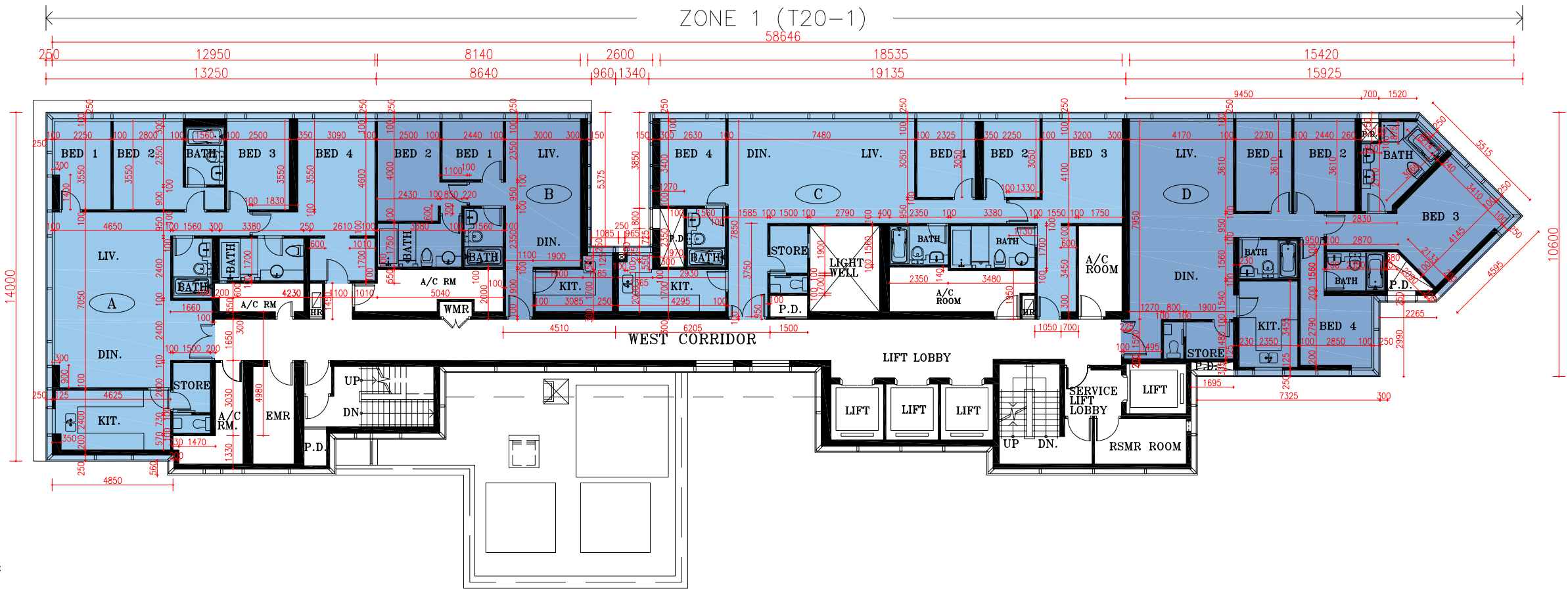
Part Plan of Flat A of 80/F. of Zone 1 of Tower 20* 第20座，第1區，80樓A室部分平面圖*
