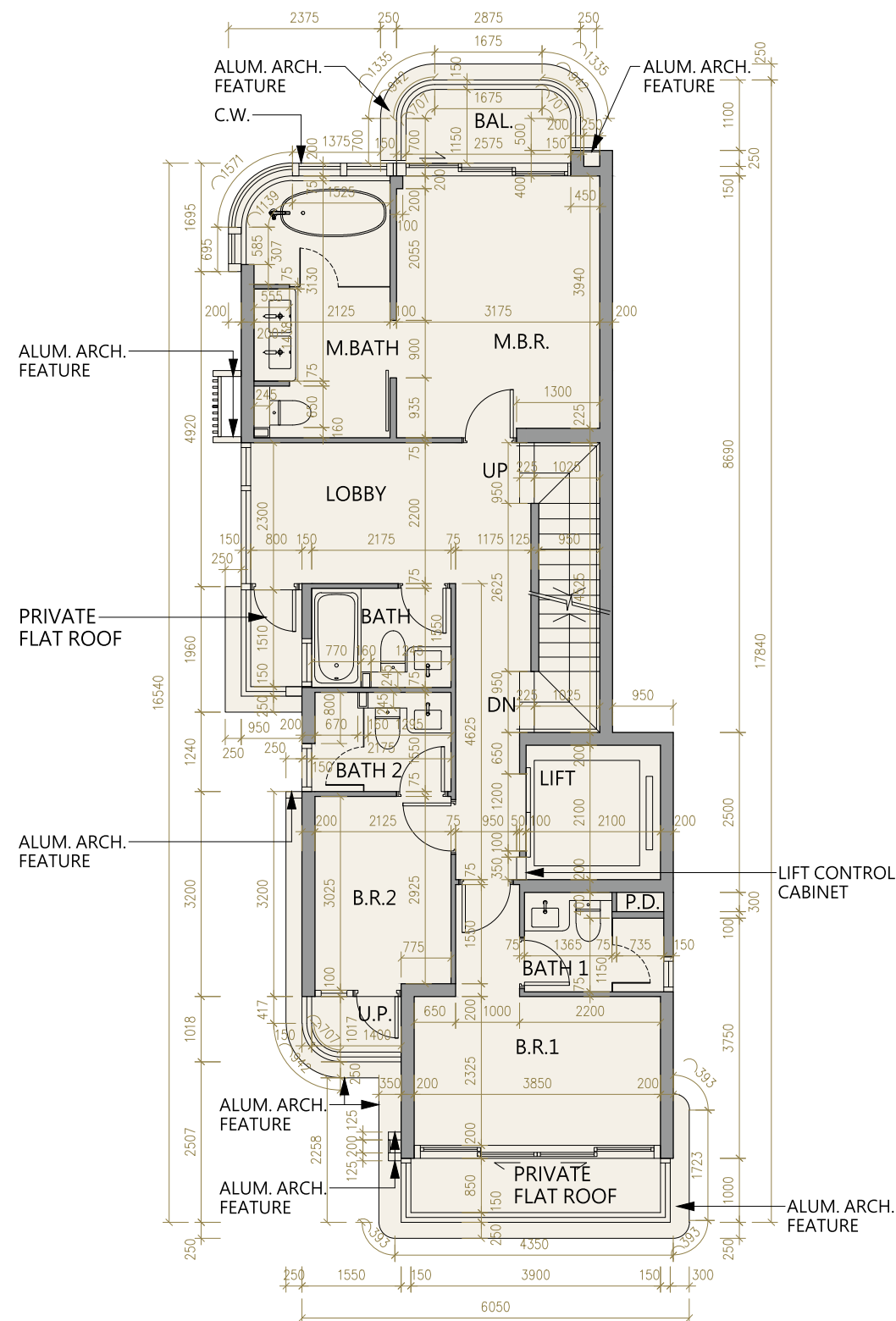
Villa 5 | 1/F & Roof Floor Plan 洋房 5 | 1樓及天台樓面平面圖
