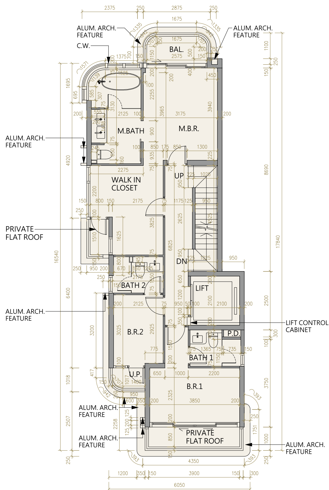
Villa 2 | 1/F & Roof Floor Plan 洋房 2 | 1樓及天台樓面平面圖
