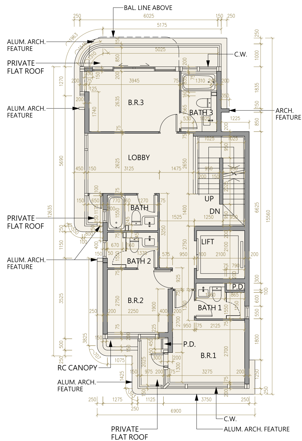
Villa 8 | 1/F, 2/F Floor Plan 洋房 8 | 1樓、2樓樓面平面圖
