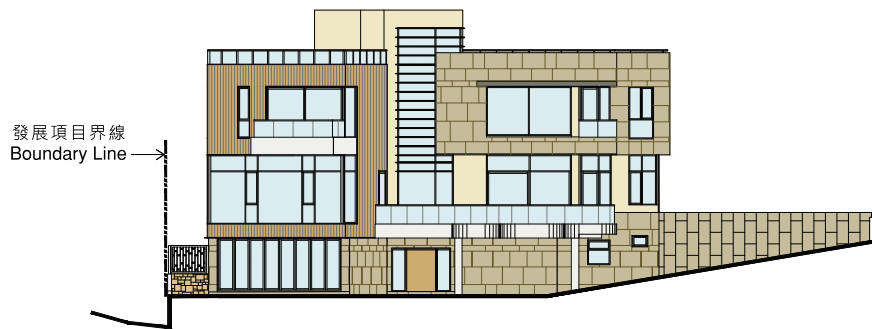
ELEVATION PLAN A 立面圖 A
