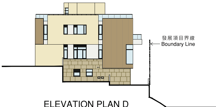
ELEVATION PLAN D 立面圖 D
