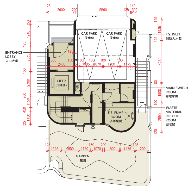
G/F 地下
