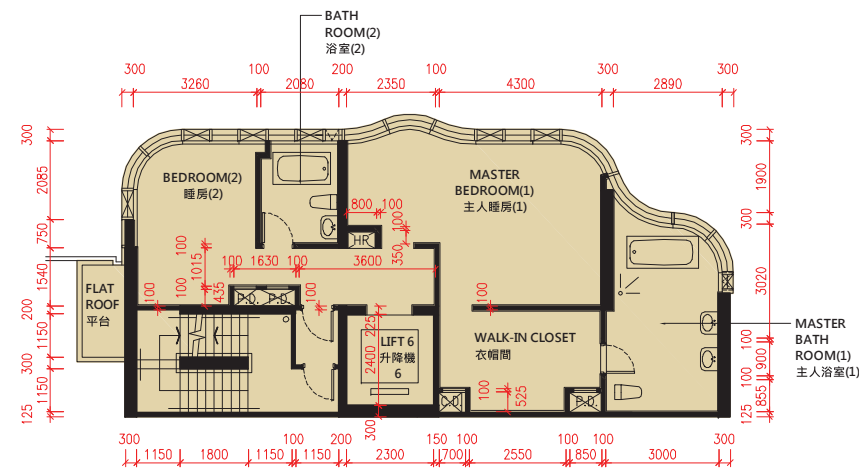
1/F 一樓
