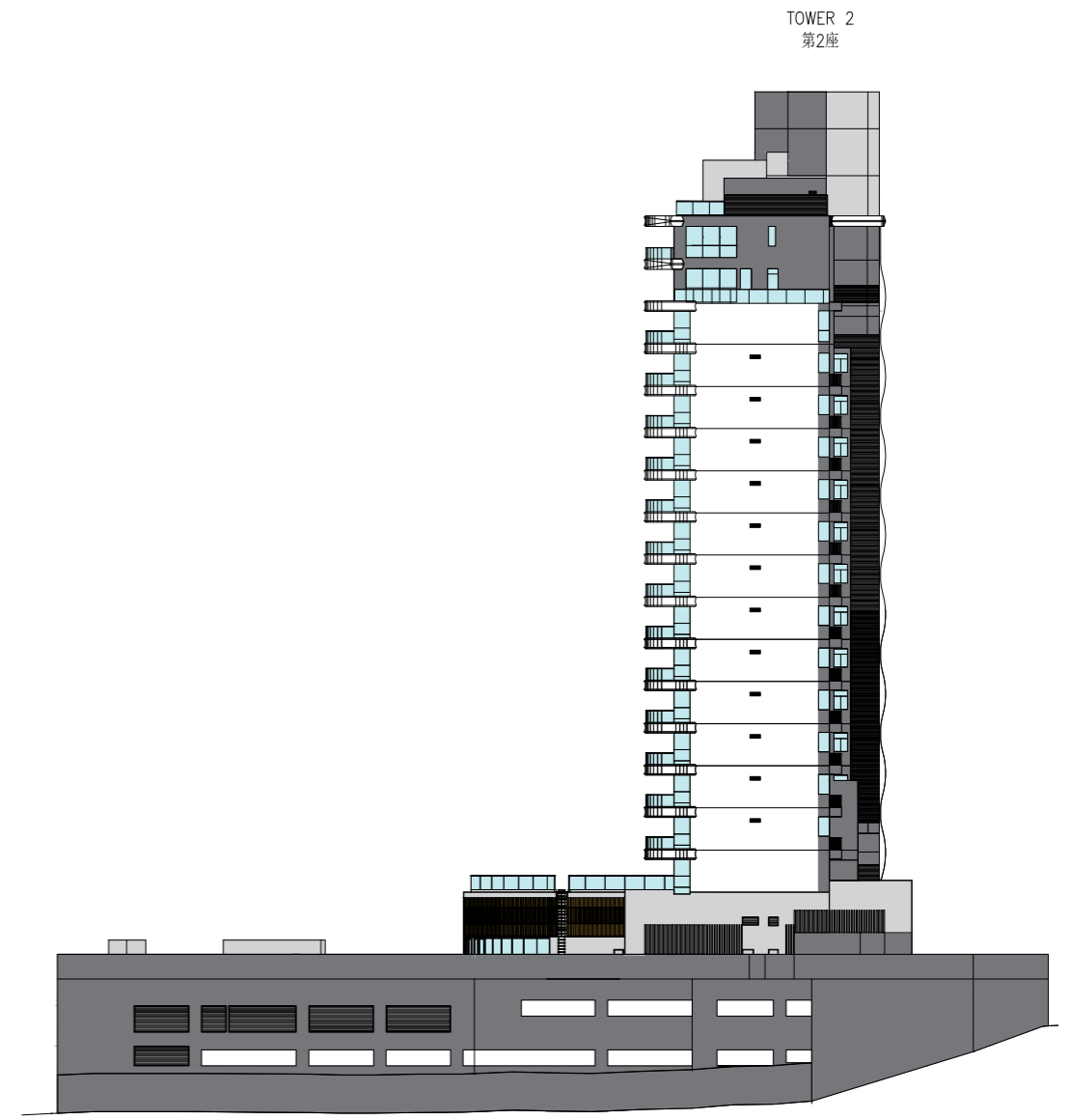
ELEVATION 2 立面 2
