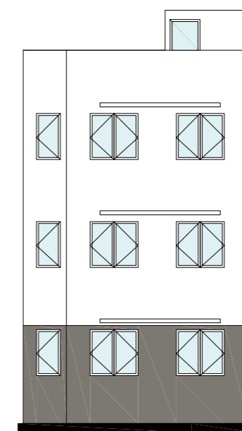
ELEVATION 3 立面圖三
