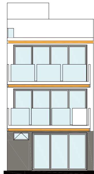
ELEVATION 1 立面圖一
