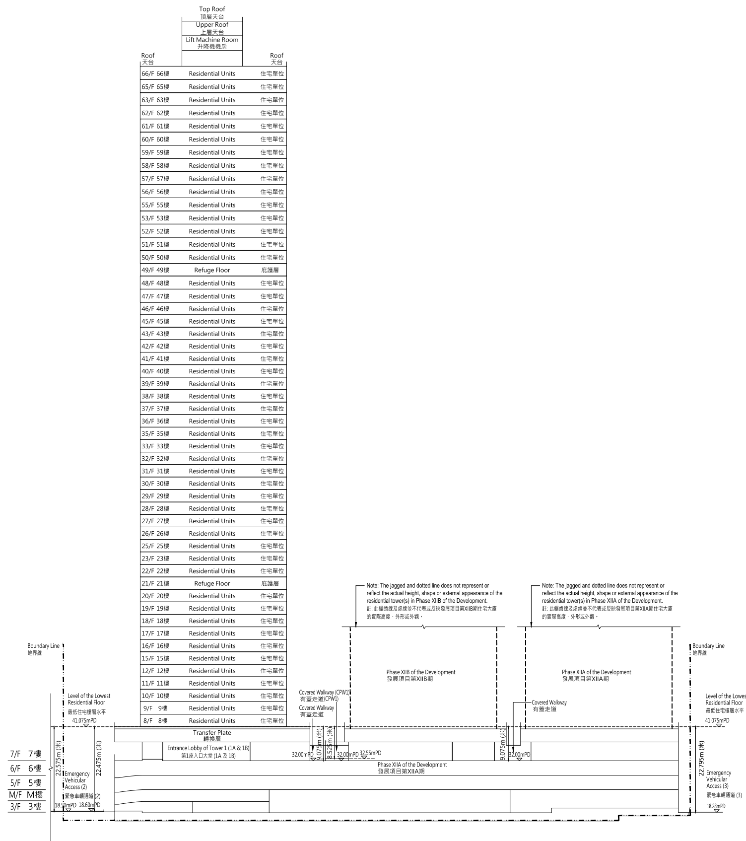
Cross-Section Plan A Tower 1 (1A & 1B) 橫截面圖 A 第1座(1A及1B)
